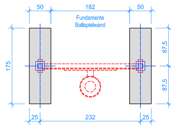
GRUNDRISS 1:50
