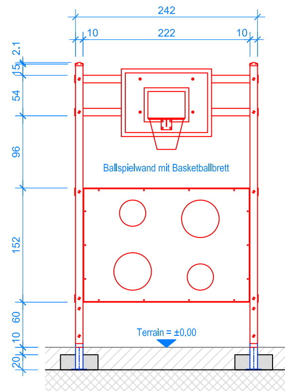
ANSICHT 1:50
