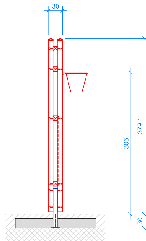
SCHNITT 1:50
