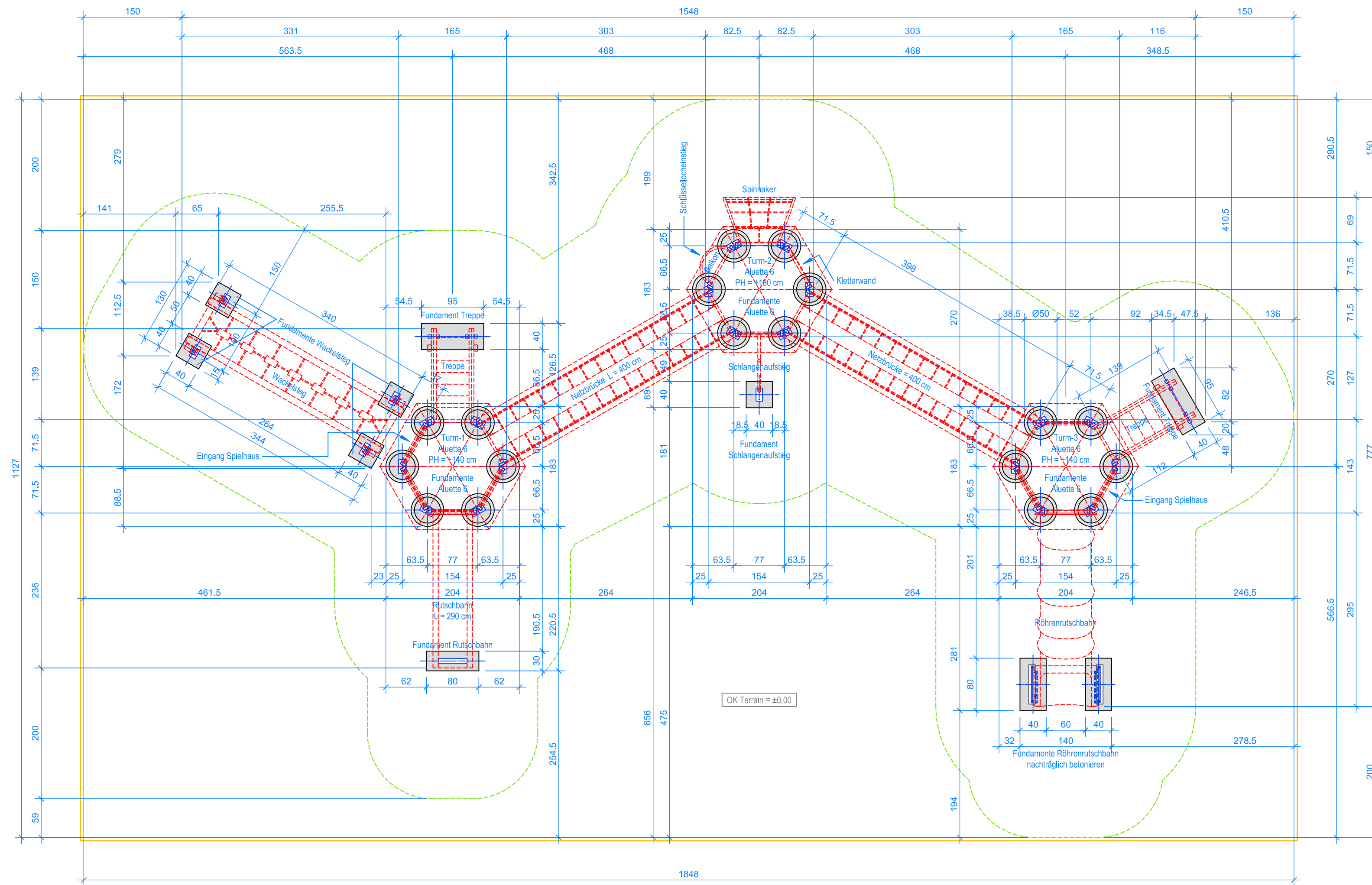
GRUNDRISS 1:50
