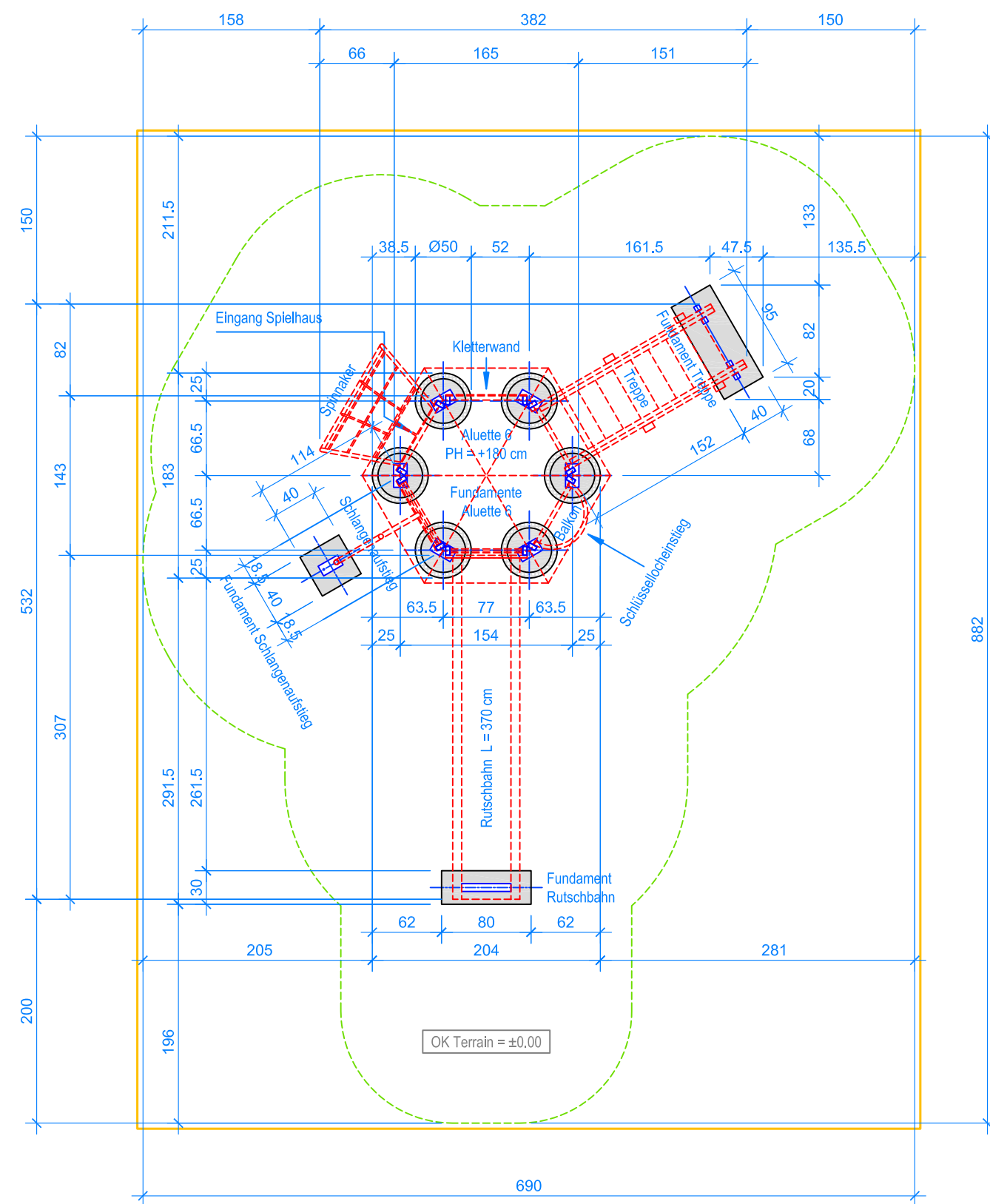
GRUNDRISS 1:50
