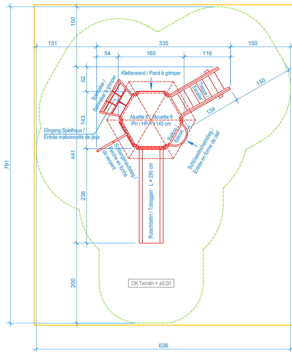
GRUNDRISS / PLAN 1:50
