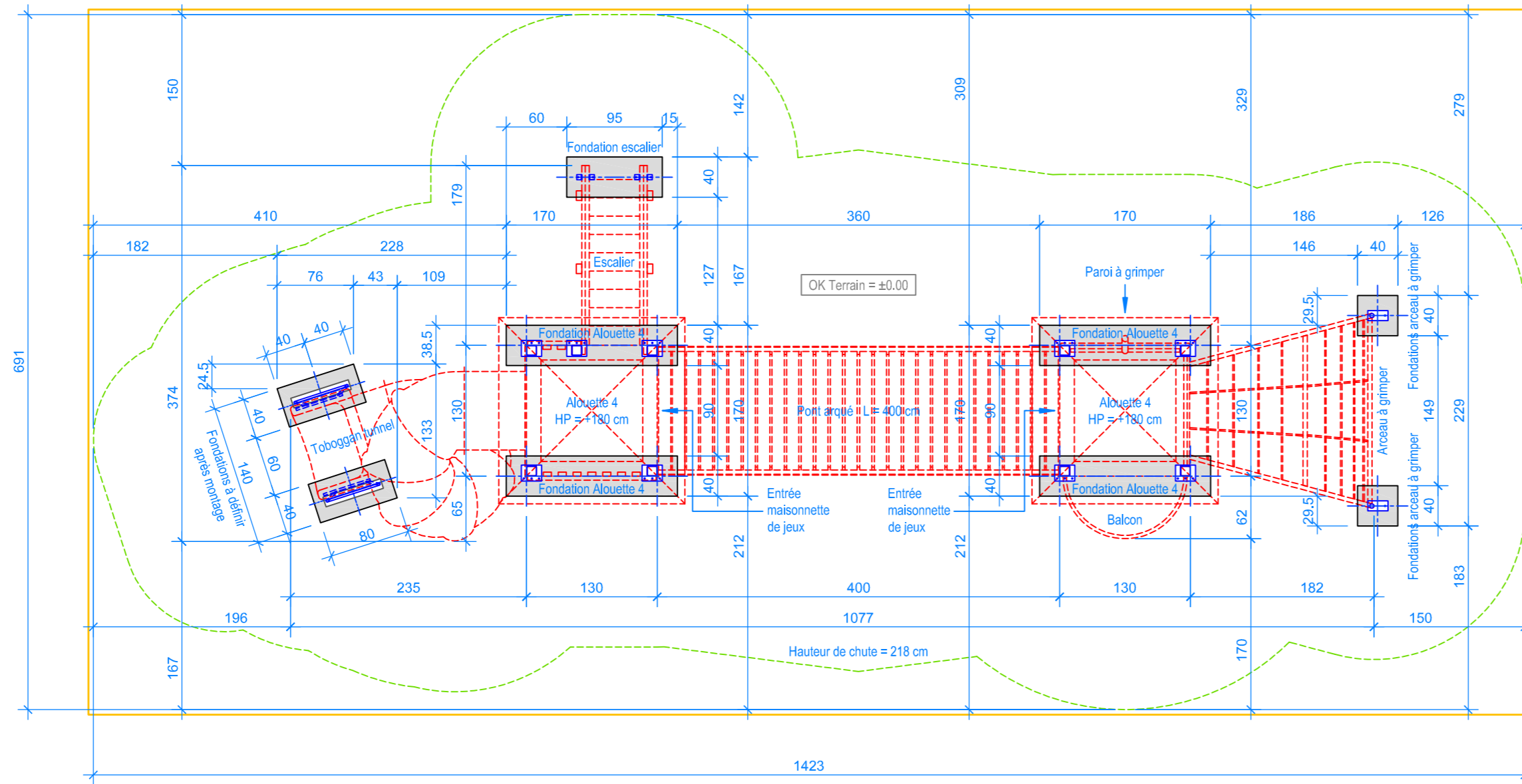
PLAN 1:50
