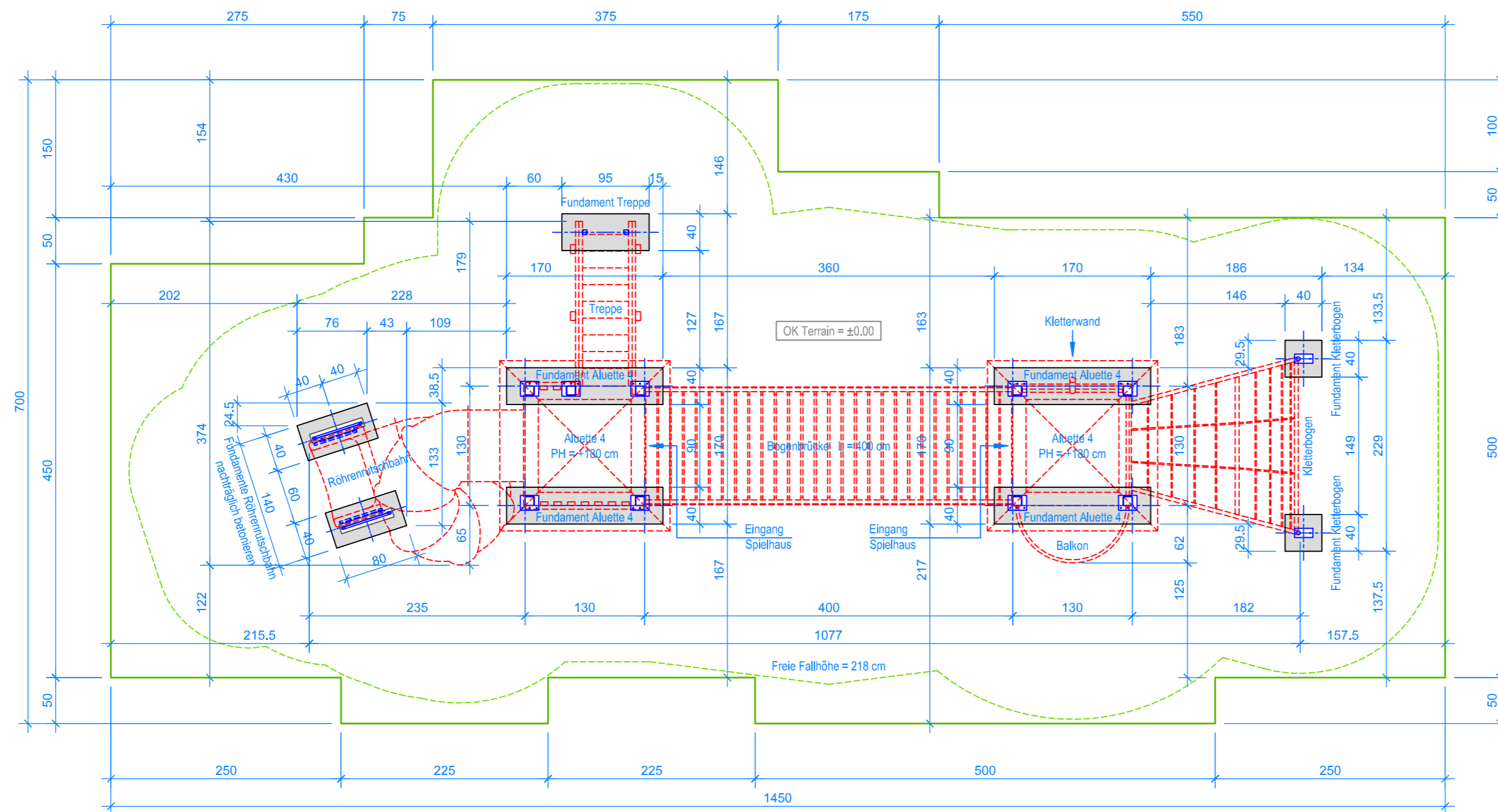
GRUNDRISS 1:50
