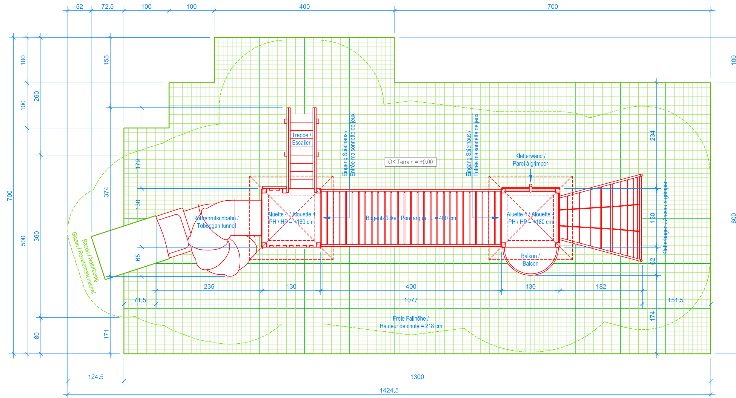
GRUNDRISS / PLAN 1:50
