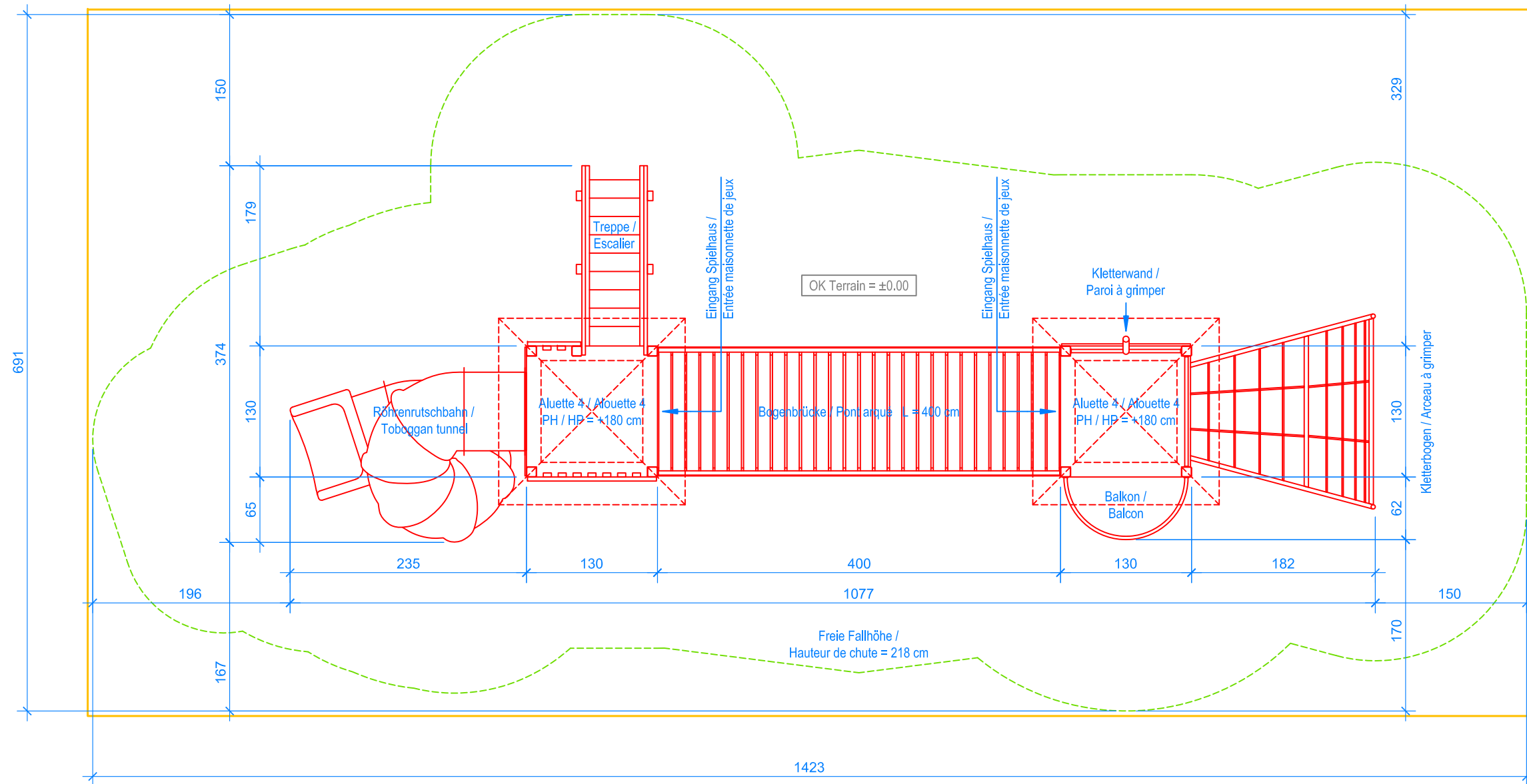
GRUNDRISS / PLAN 1:50
