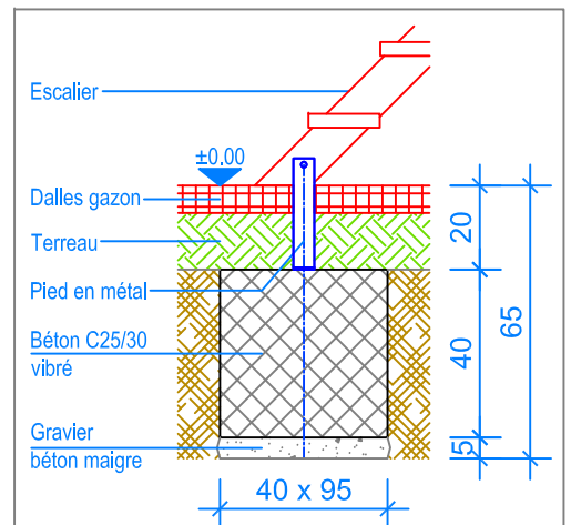
COUPE 1:20 FONDATION ESCALIER
