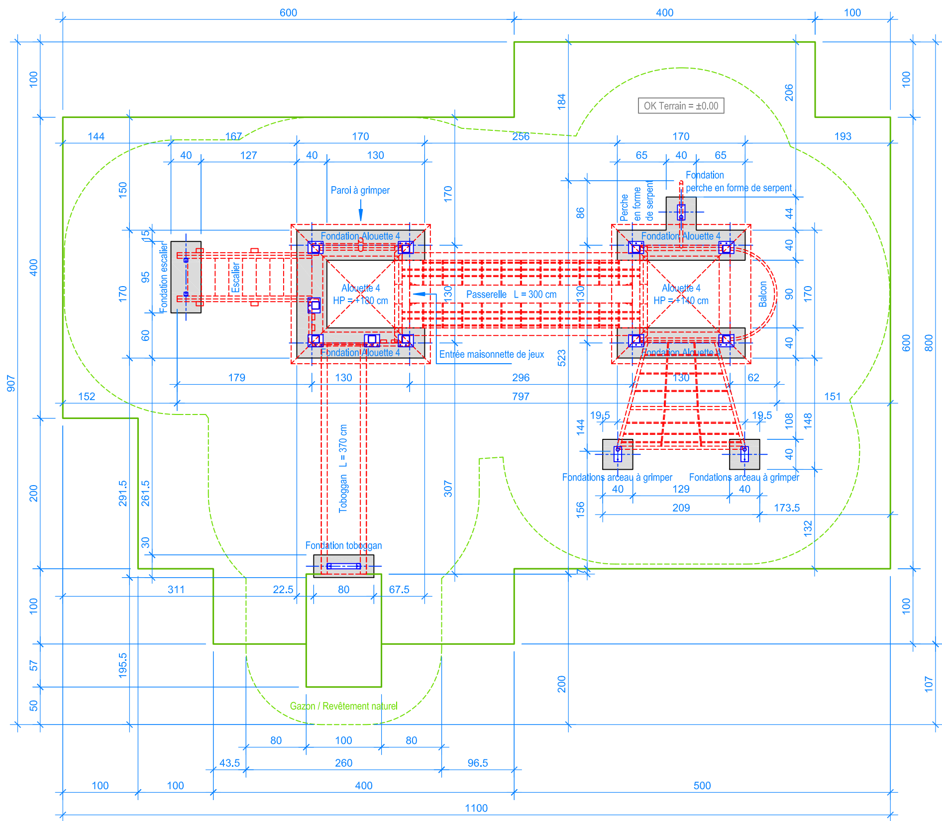
PLAN 1:50
