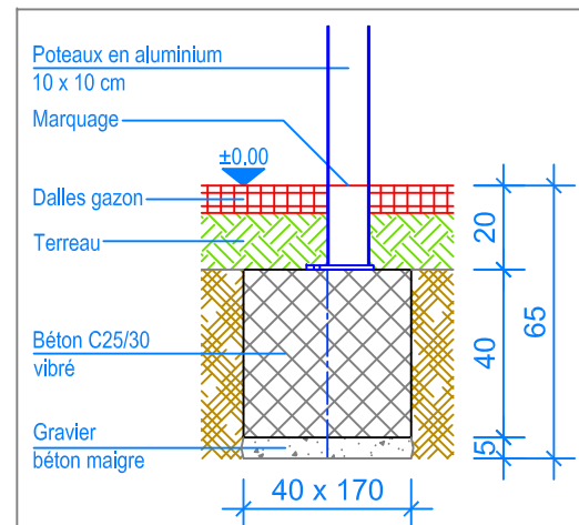
COUPE 1:20 FONDATION ALOUETTE 4
