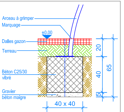
COUPE 1:20 FONDATION ARCEAU À GRIMPER
