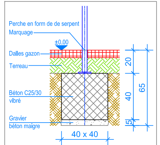
COUPE 1:20 PERCHE EN FORME DE SERPENT
