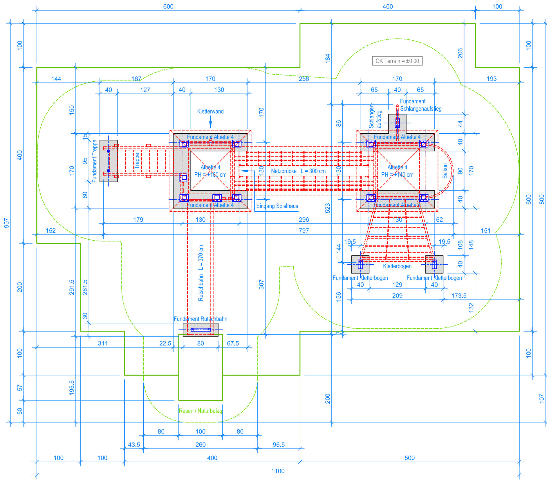
GRUNDRISS 1:50
