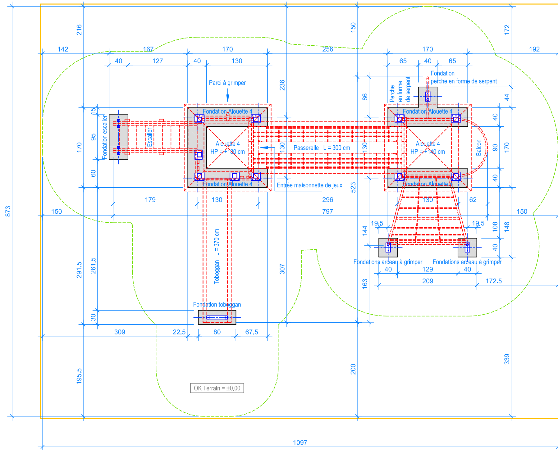
PLAN 1:50
