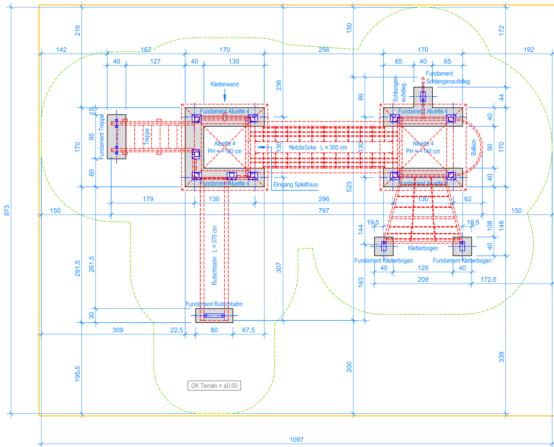
GRUNDRISS 1:50
