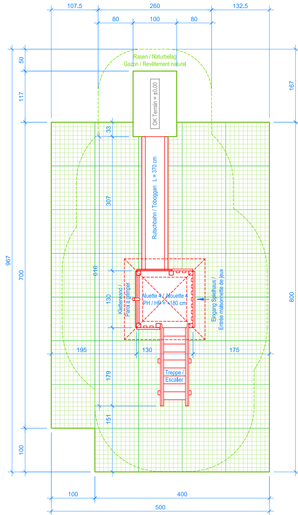
GRUNDRISS / PLAN 1:50
