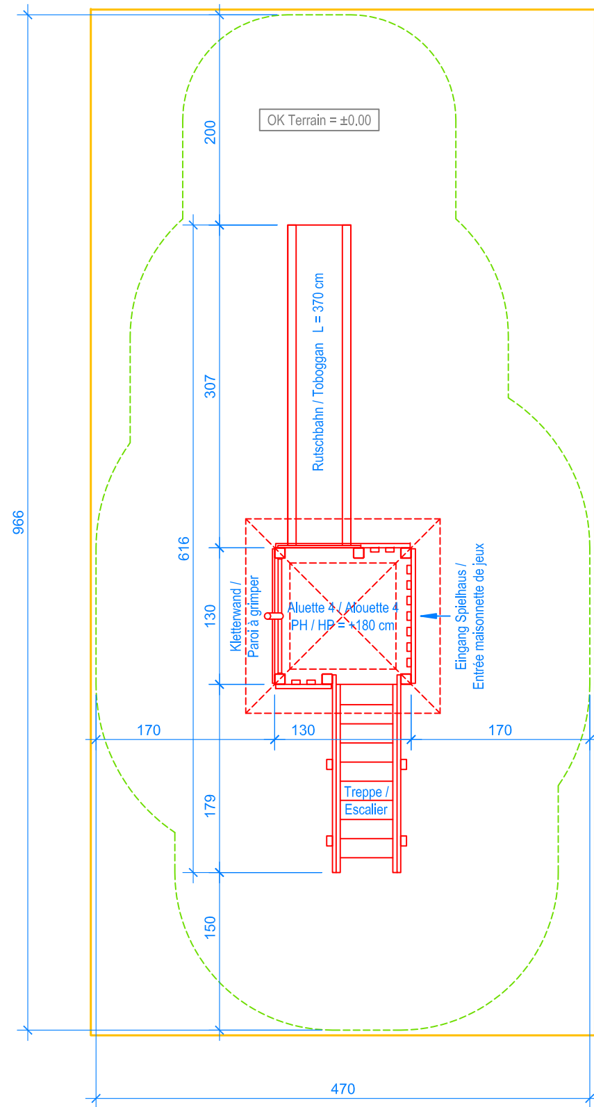
GRUNDRISS / PLAN 1:50
