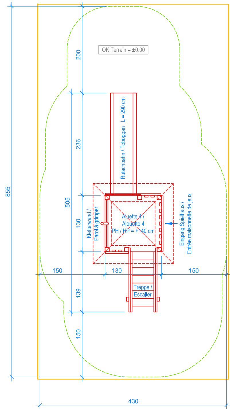
GRUNDRISS / PLAN 1:50
