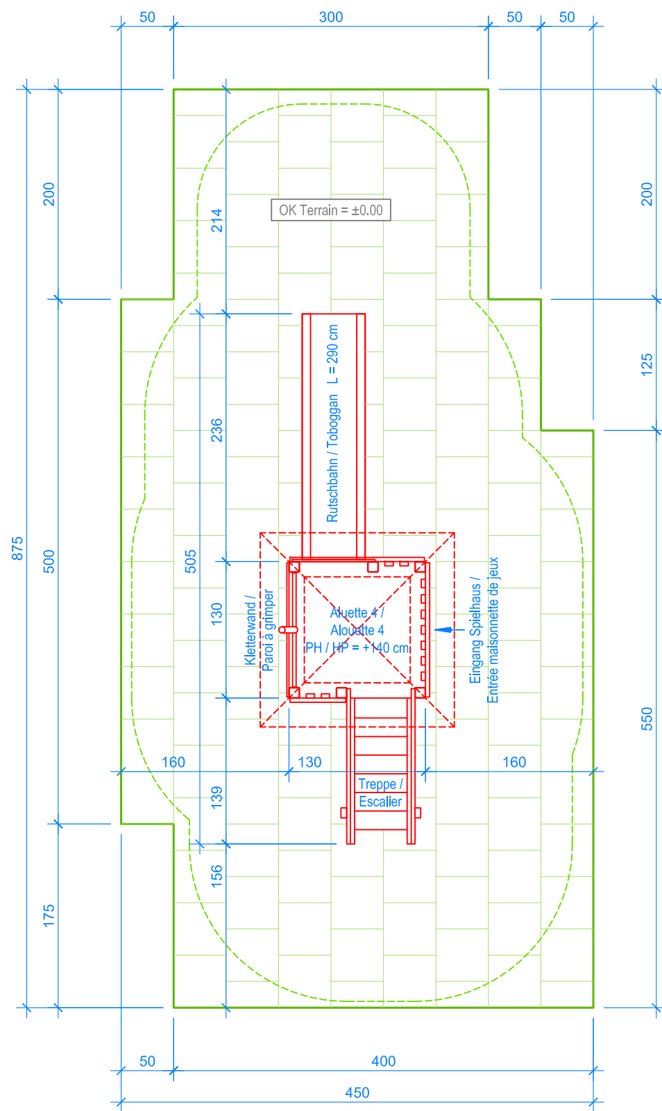
GRUNDRISS / PLAN 1:50
