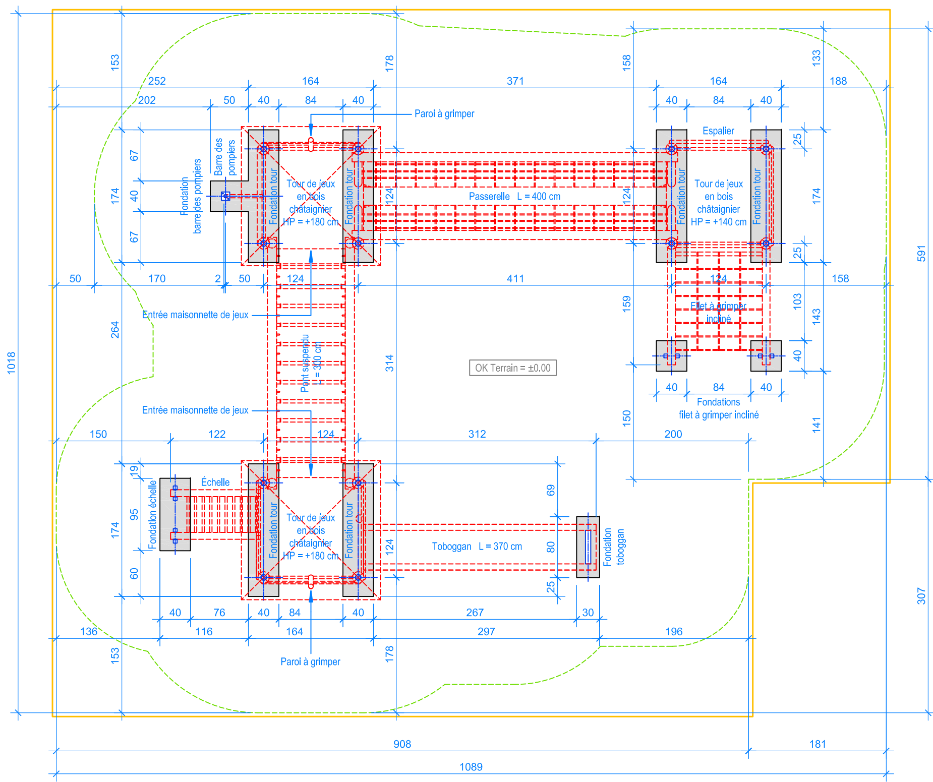
PLAN 1:50
