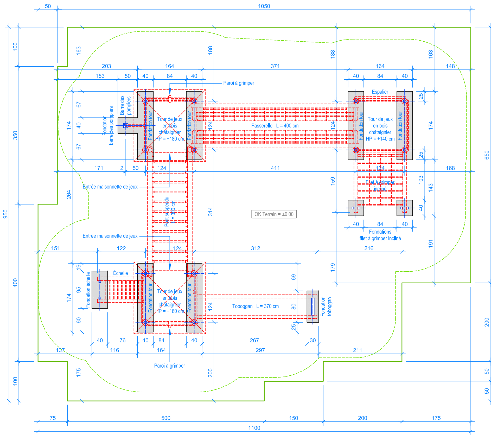
PLAN 1:50
