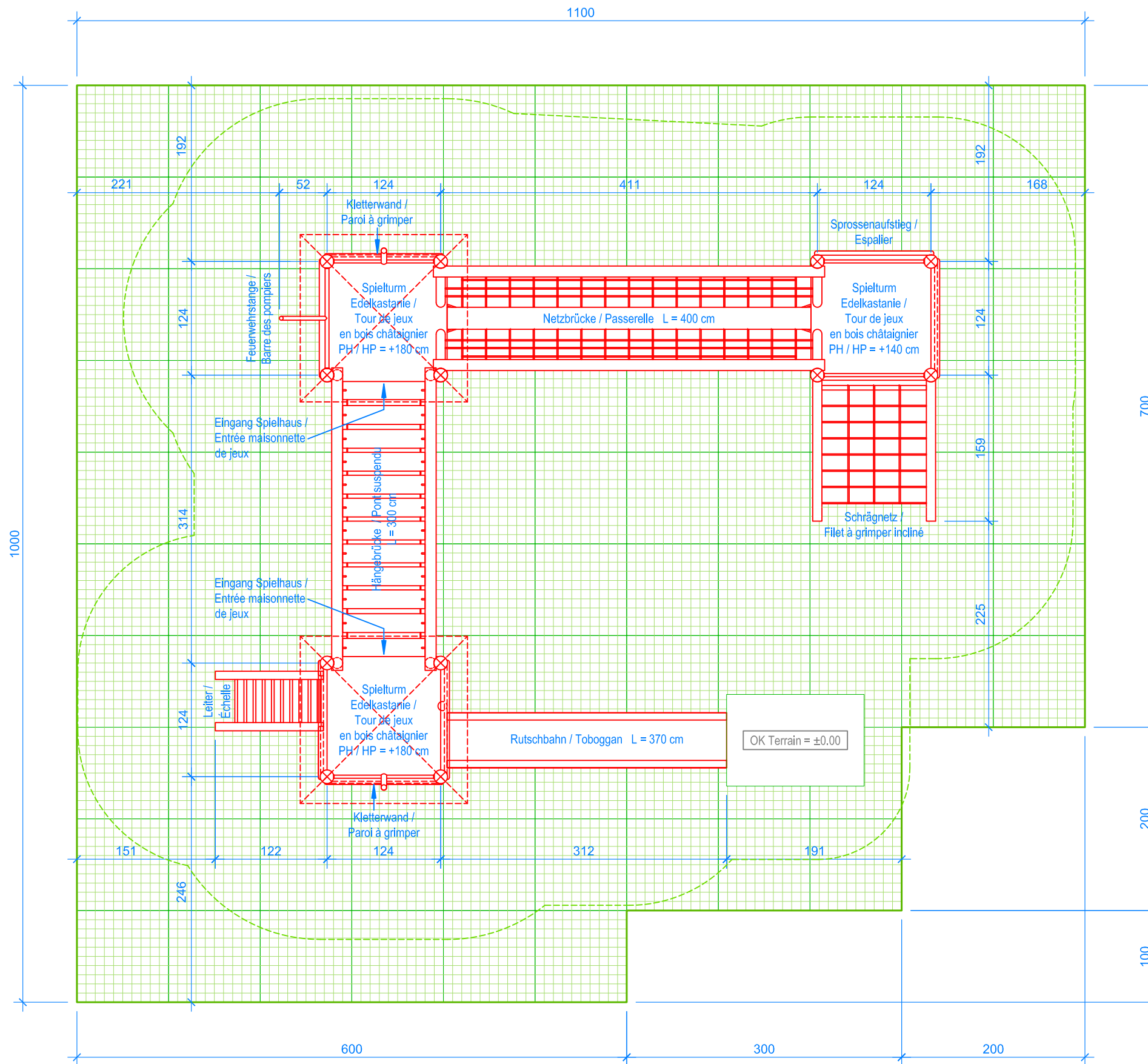
GRUNDRISS / PLAN 1:50
