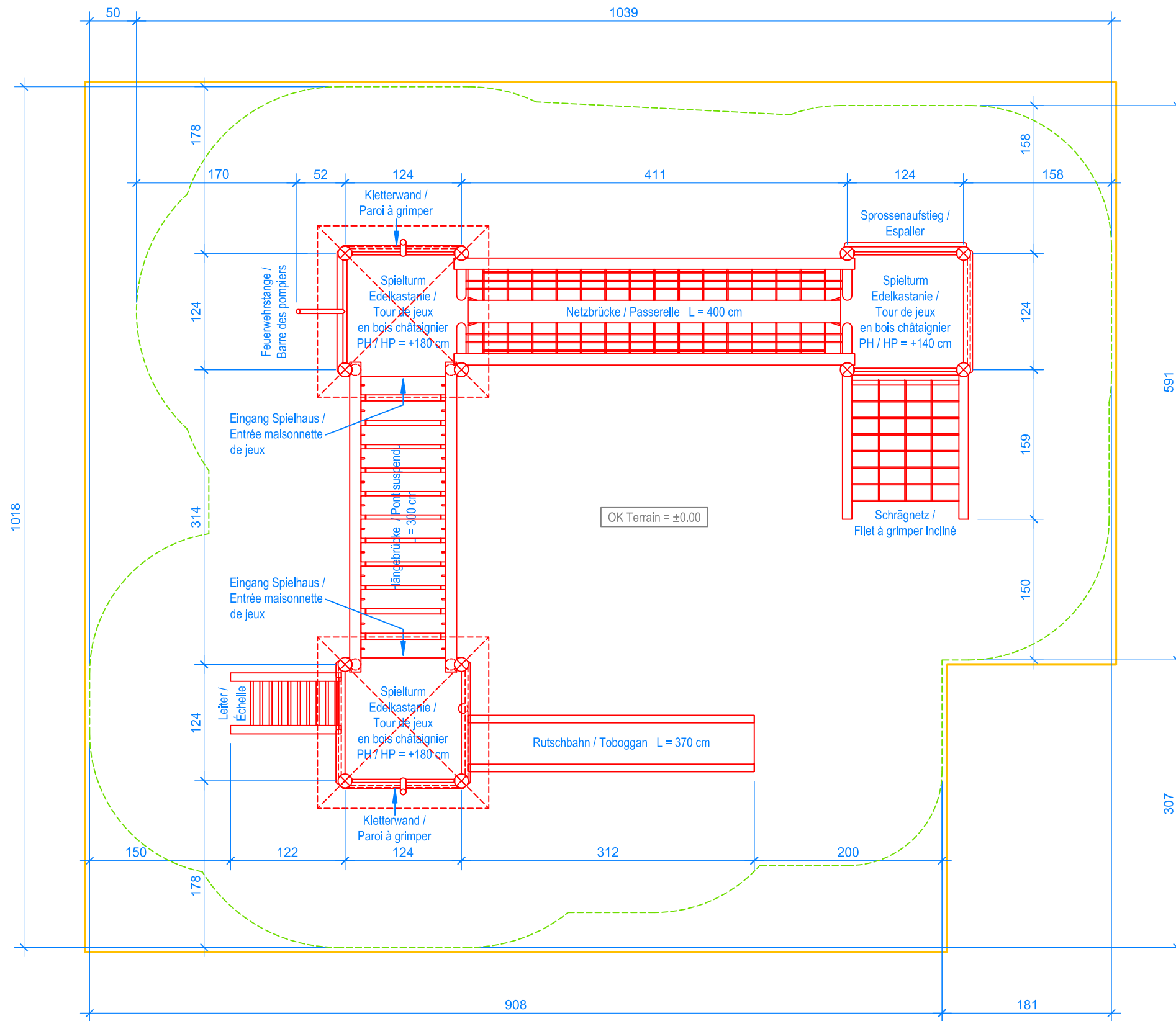
GRUNDRISS / PLAN 1:50
