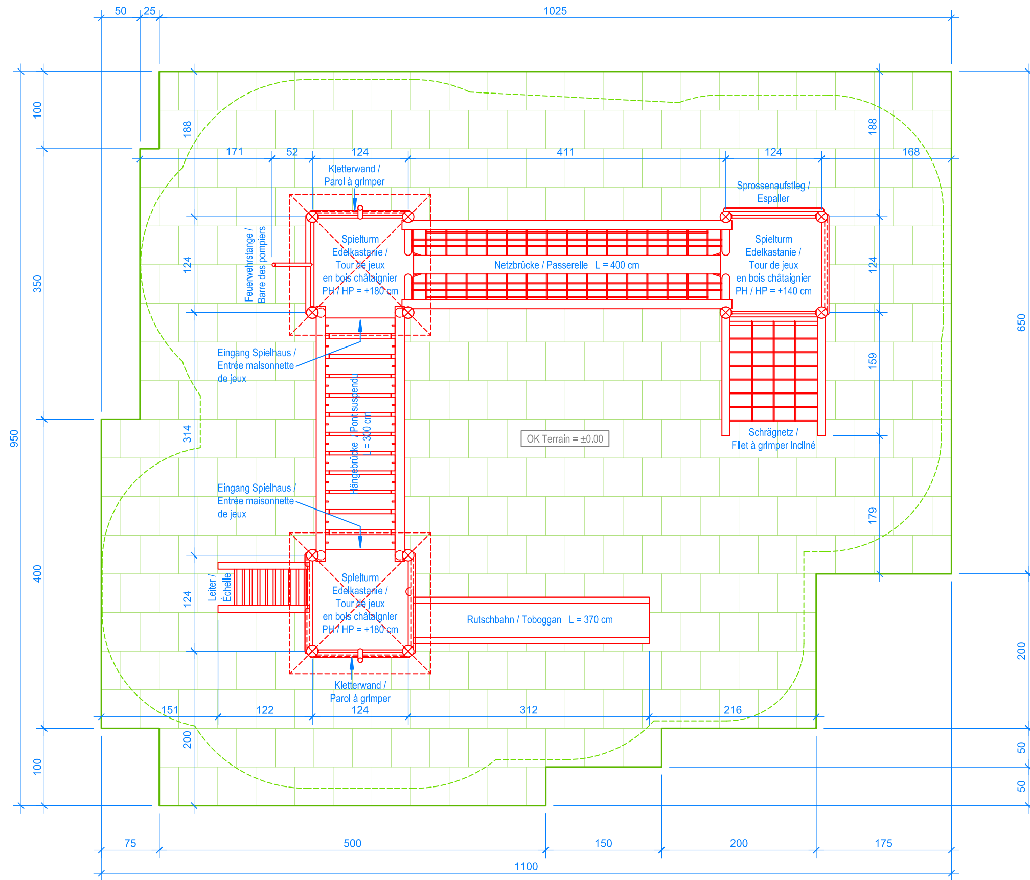
GRUNDRISS / PLAN 1:50
