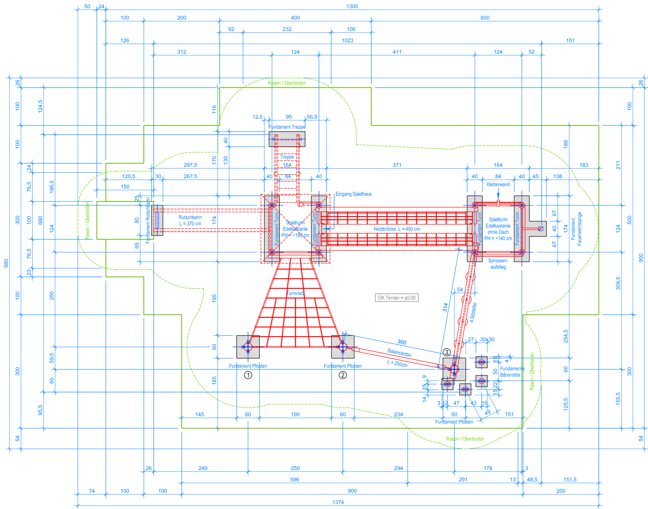
GRUNDRISS 1:50
