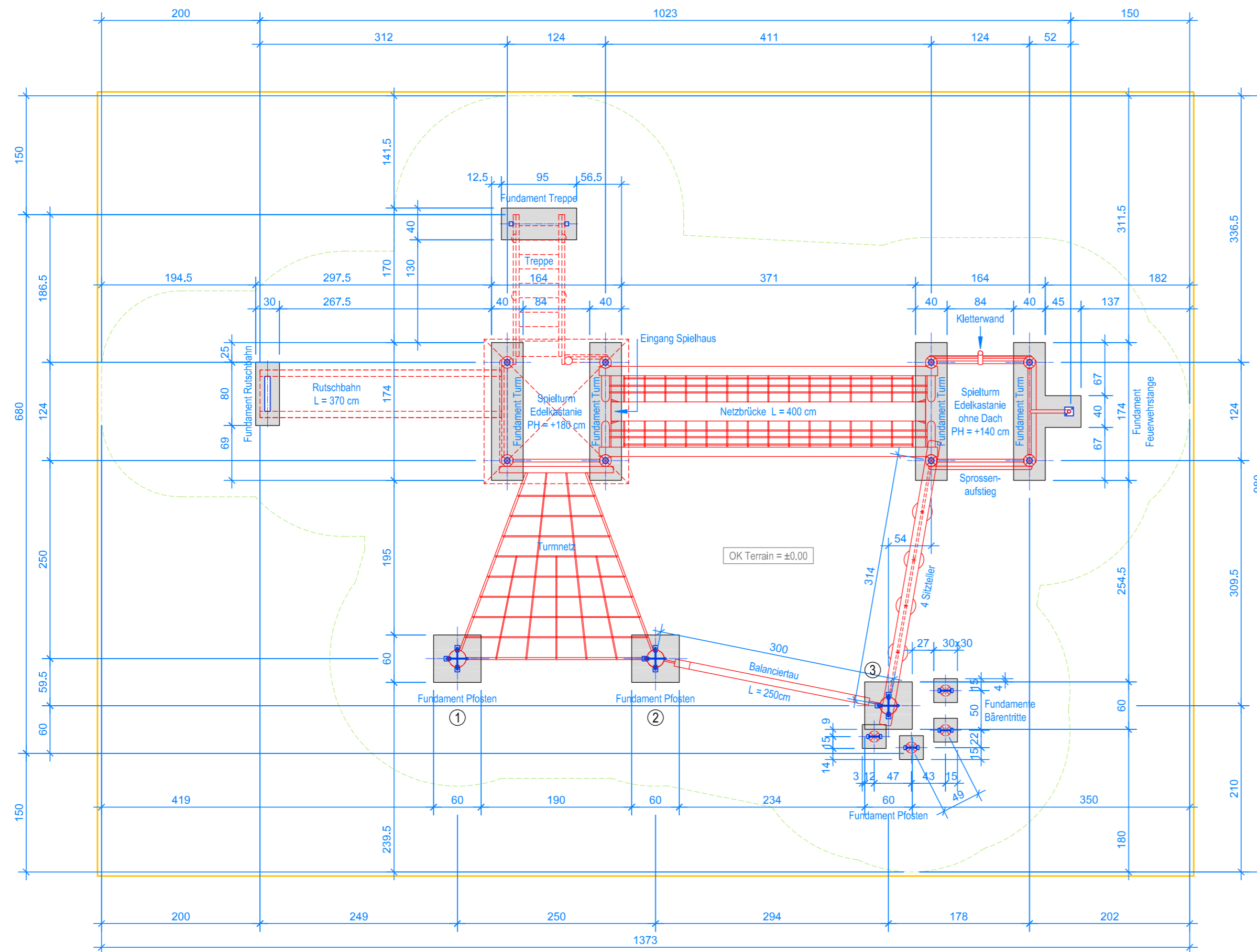
GRUNDRISS 1:50
