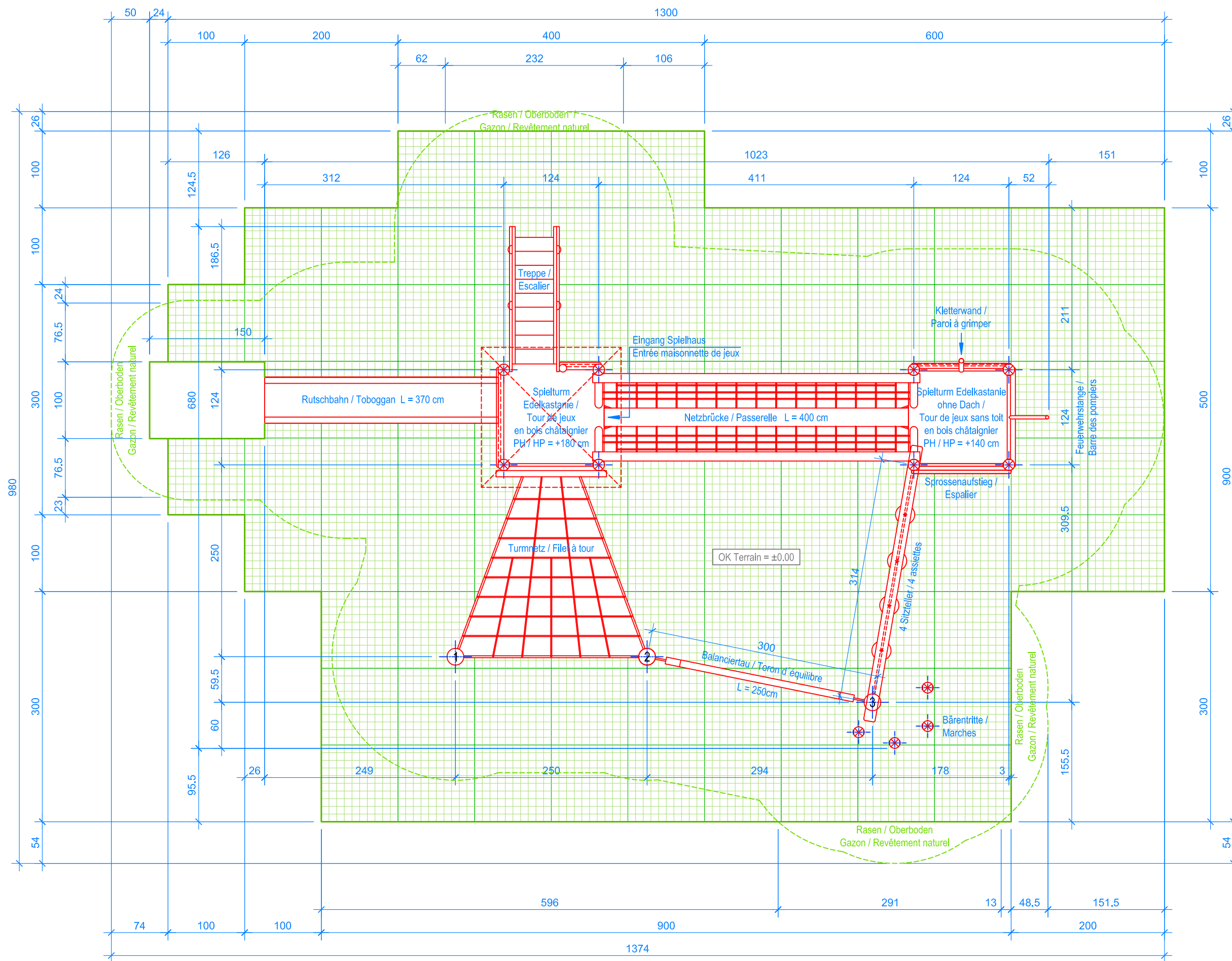
GRUNDRISS / PLAN 1:50
