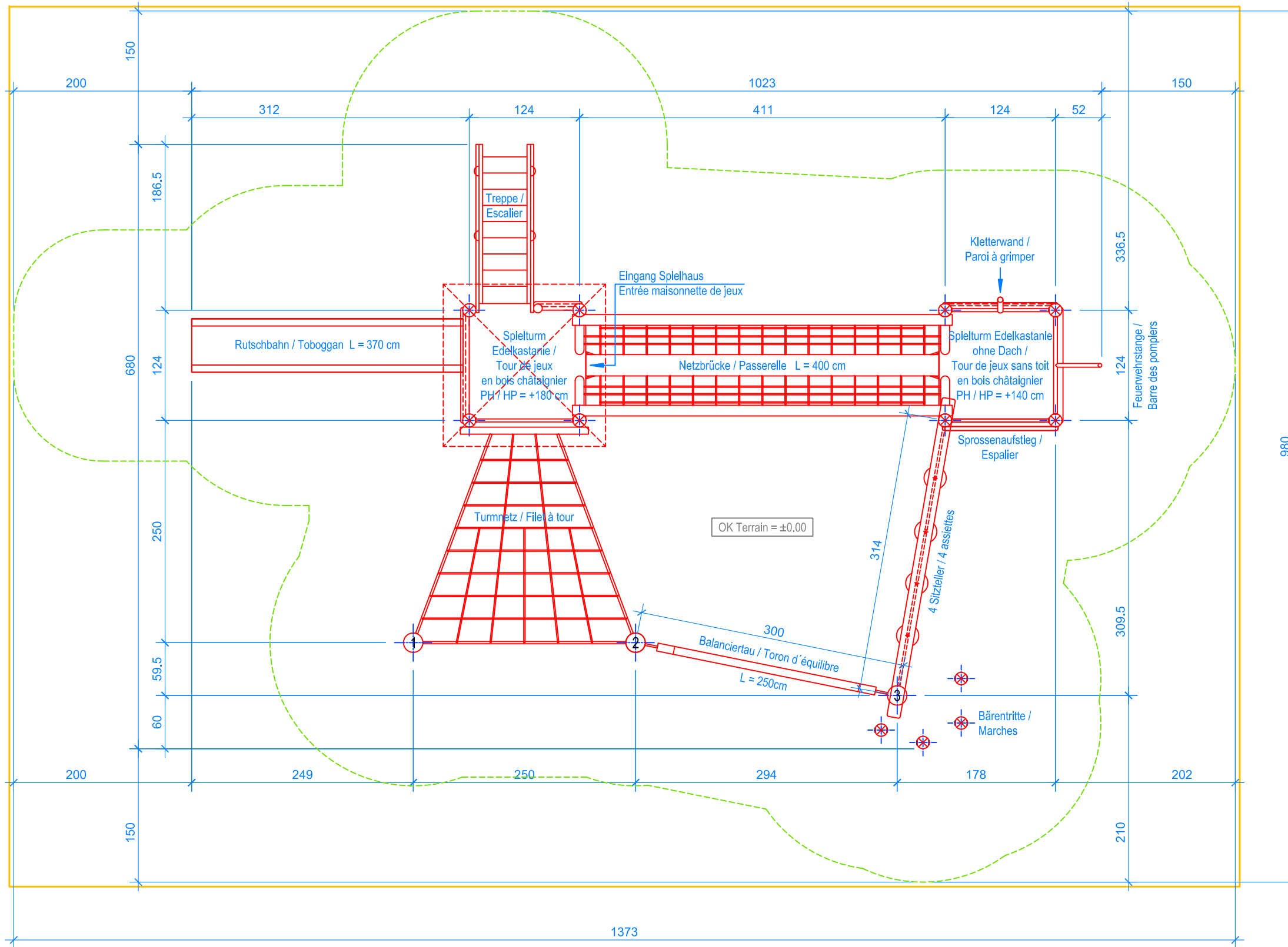
GRUNDRISS / PLAN 1:50
