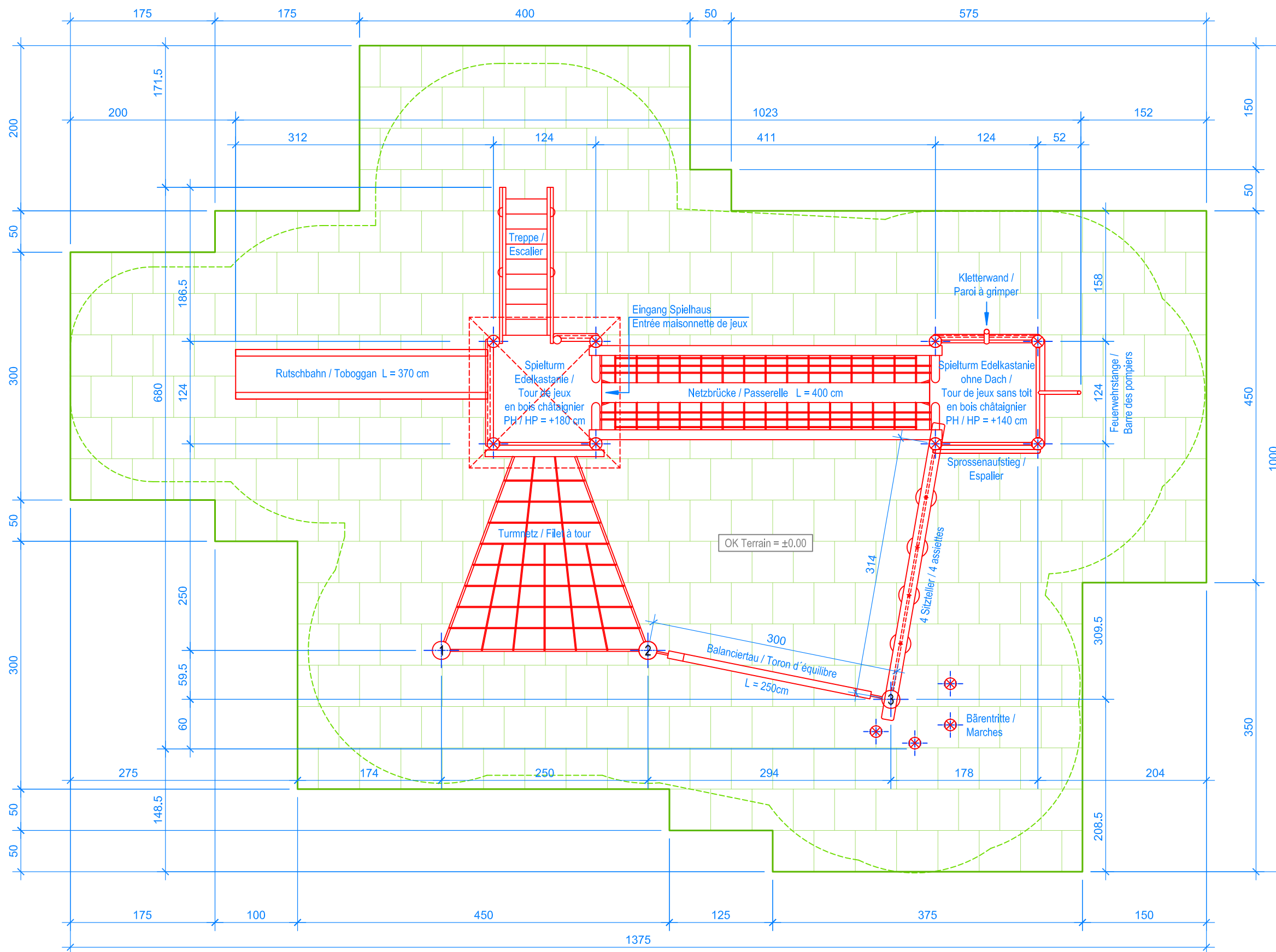
GRUNDRISS / PLAN 1:50
