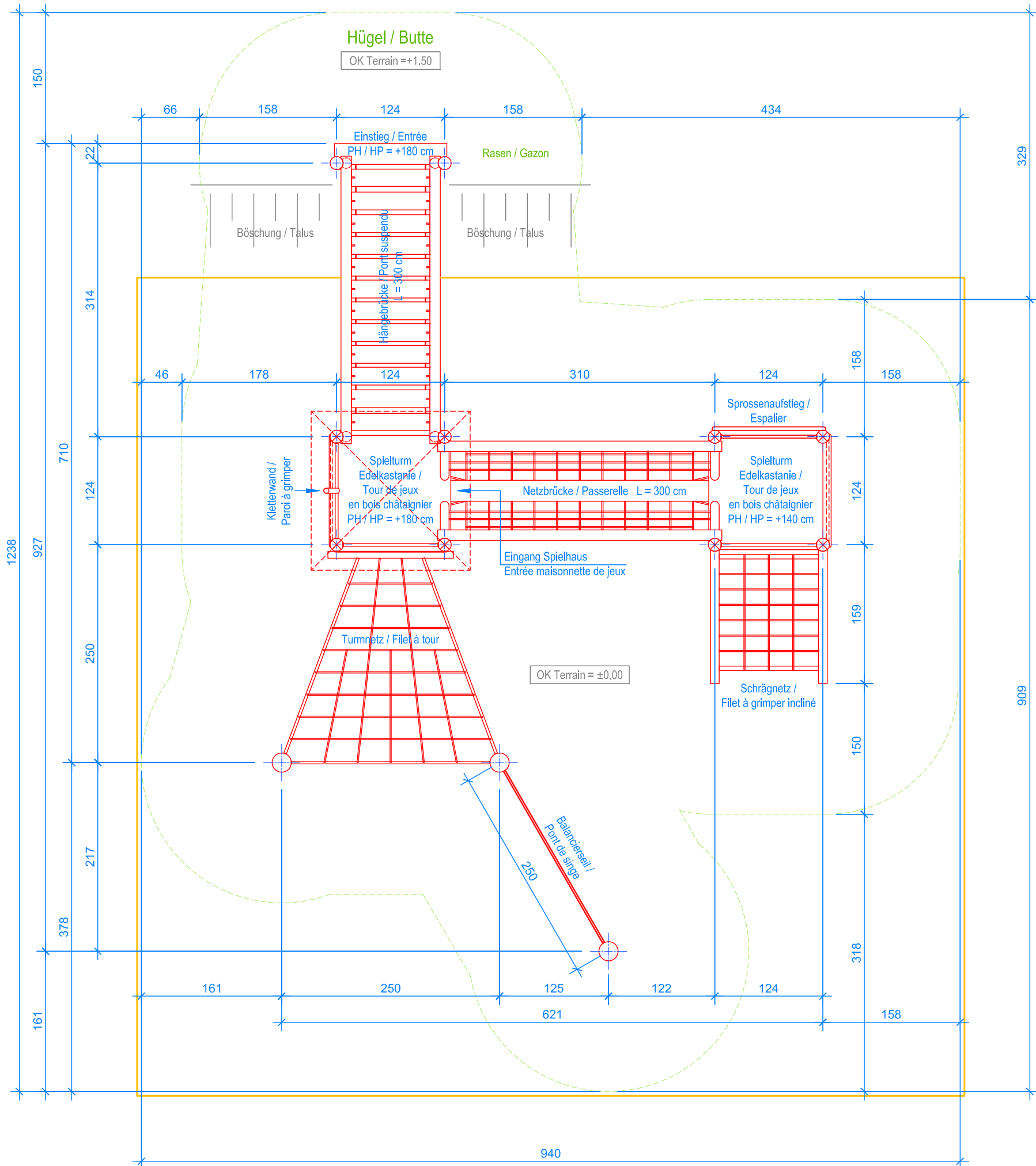
GRUNDRISS / PLAN 1:50
