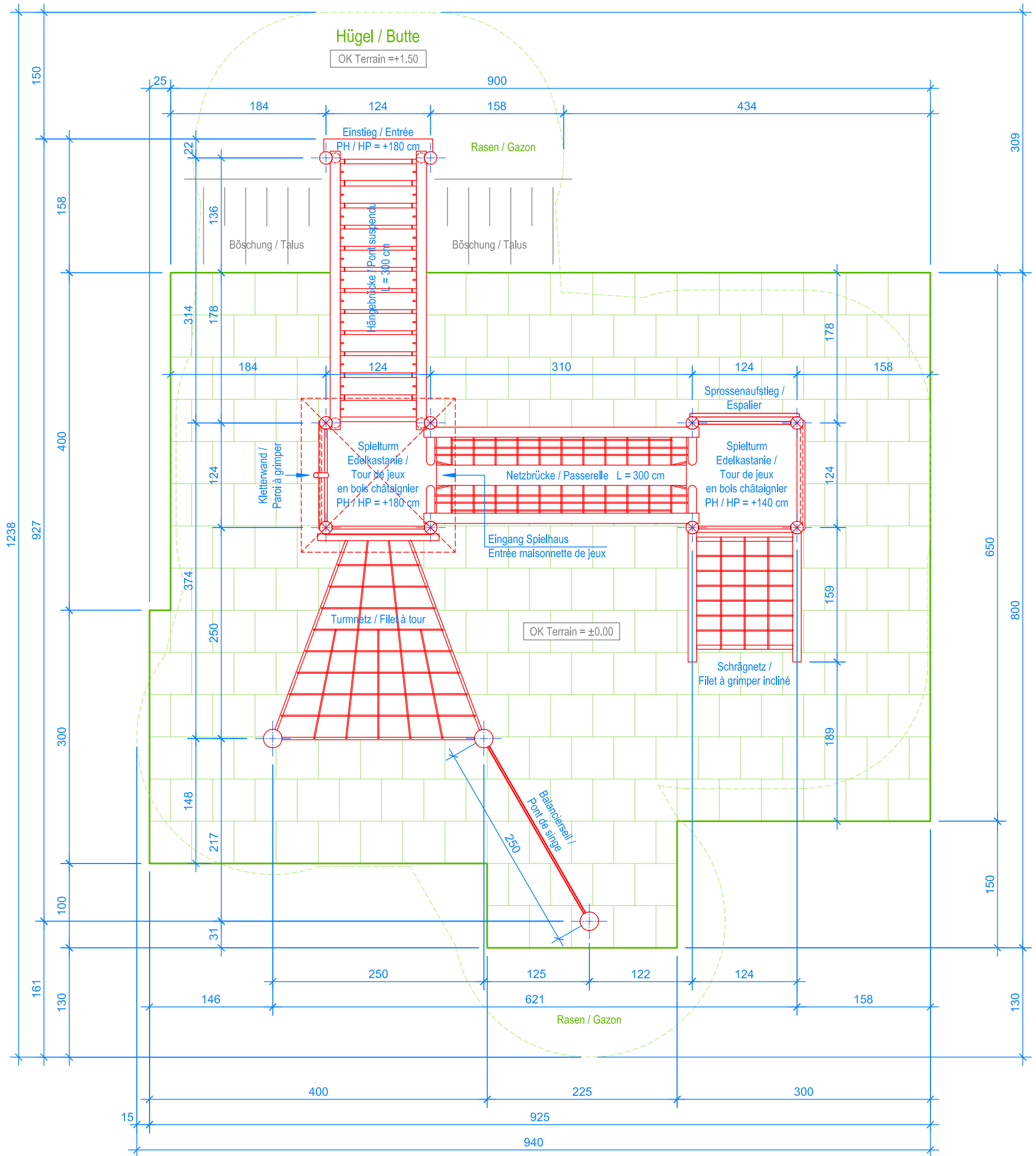
GRUNDRISS / PLAN 1:50
