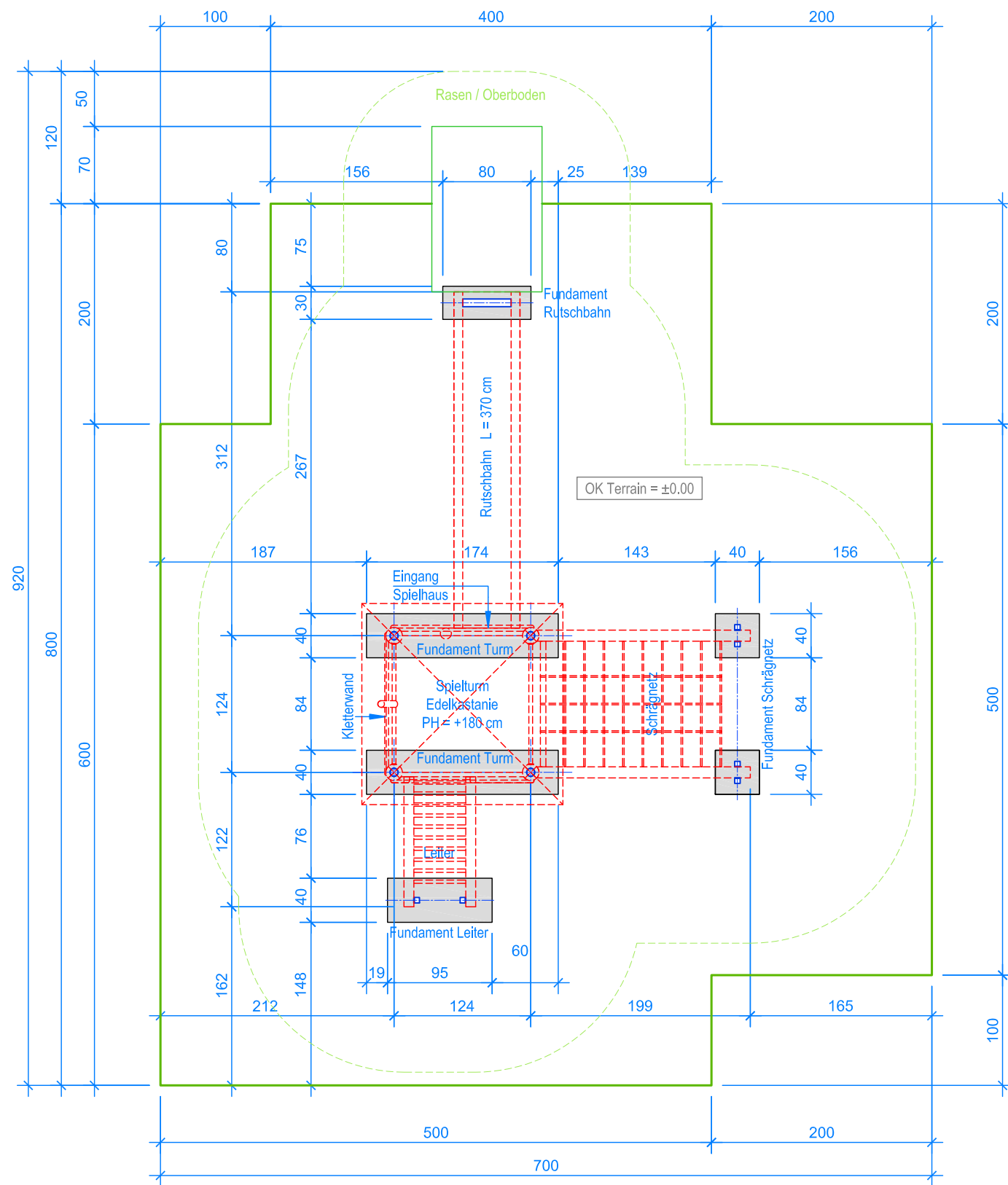
GRUNDRISS 1:50
