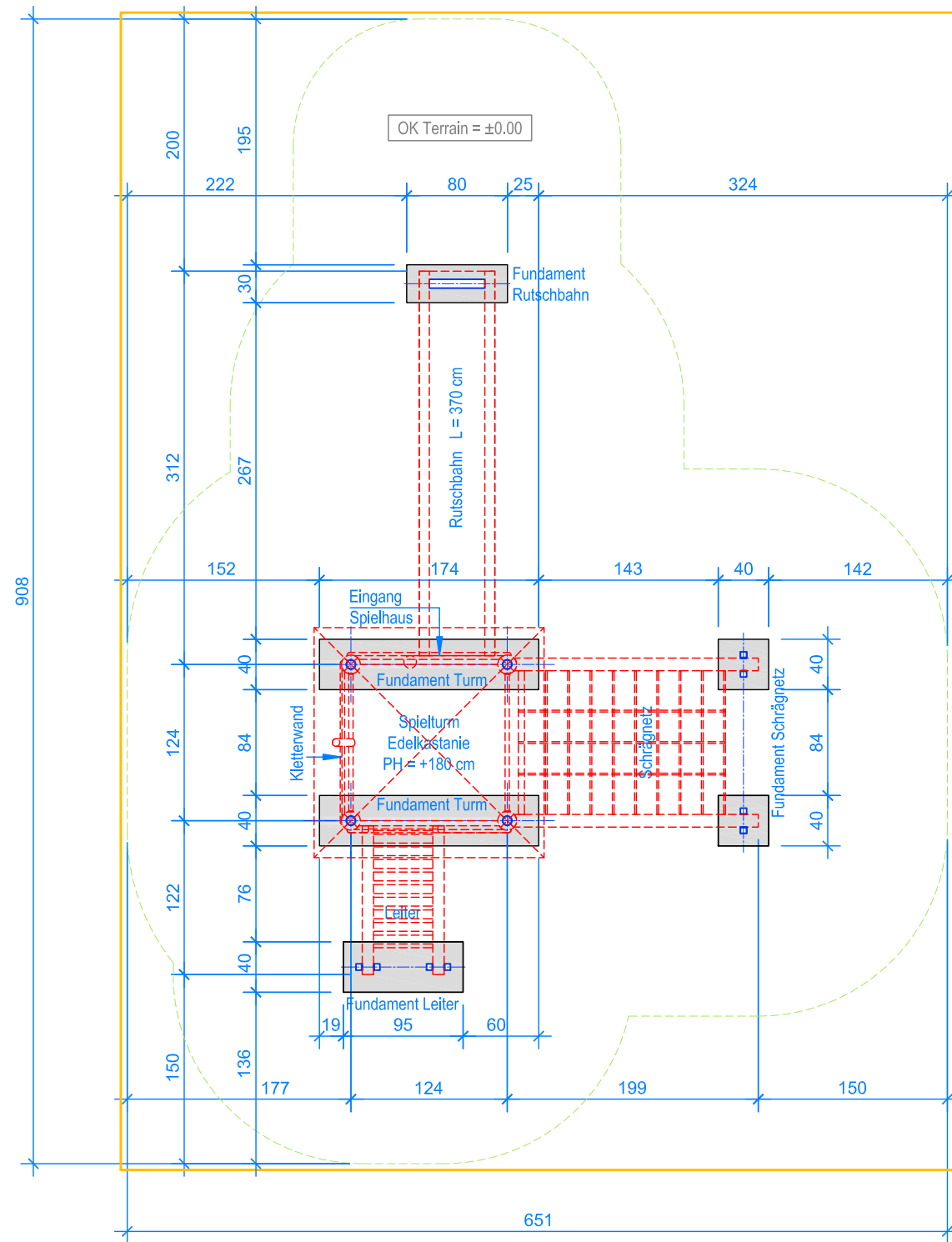
GRUNDRISS 1:50
