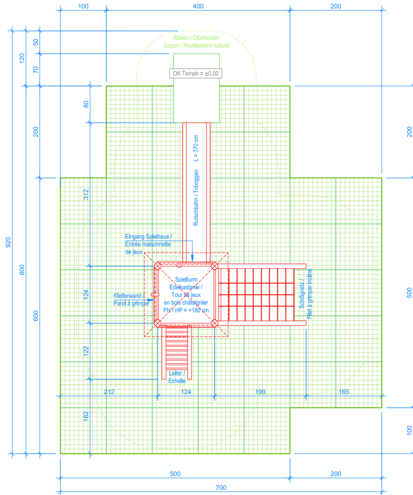
GRUNDRISS / PLAN 1:50
