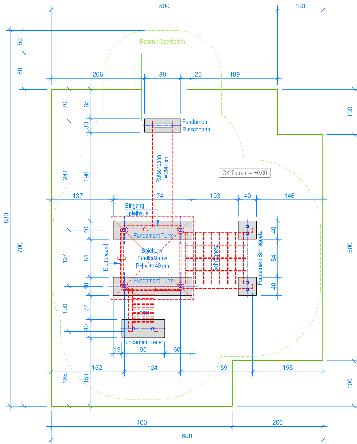
GRUNDRISS 1:50
