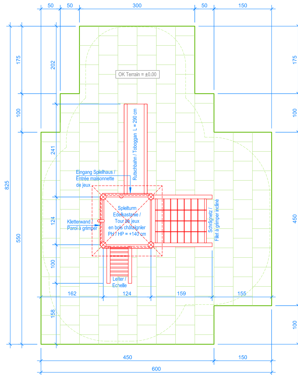
GRUNDRISS / PLAN 1:50
