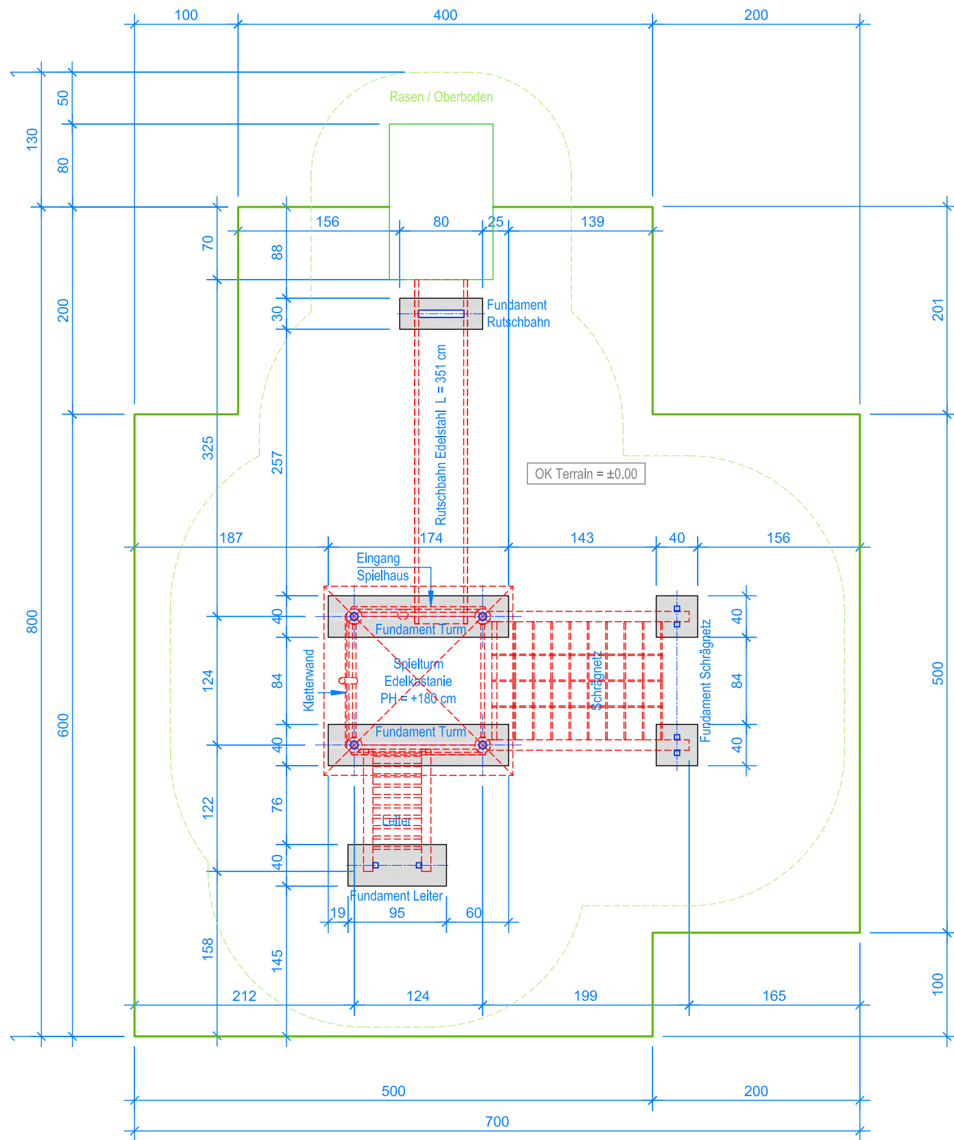
GRUNDRISS 1:50
