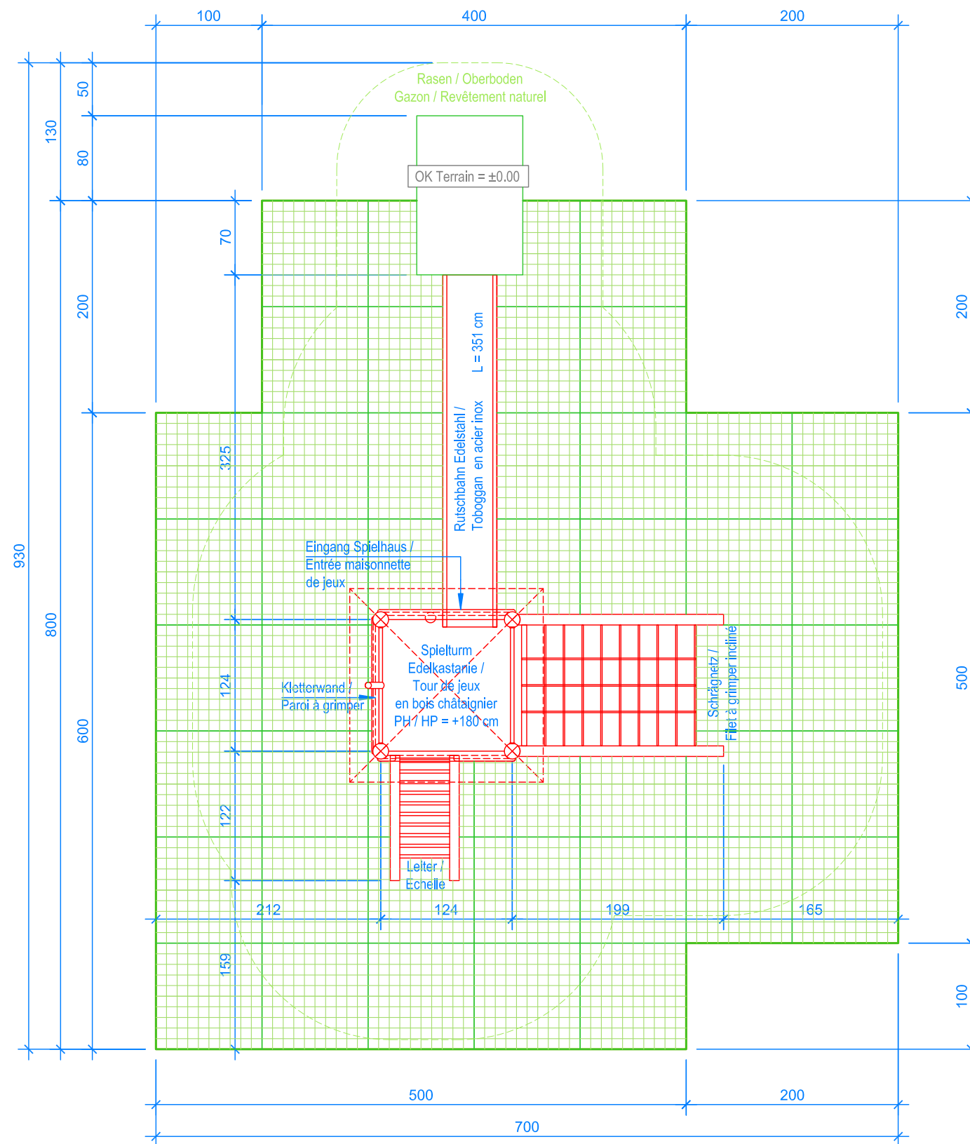
GRUNDRISS / PLAN 1:50
