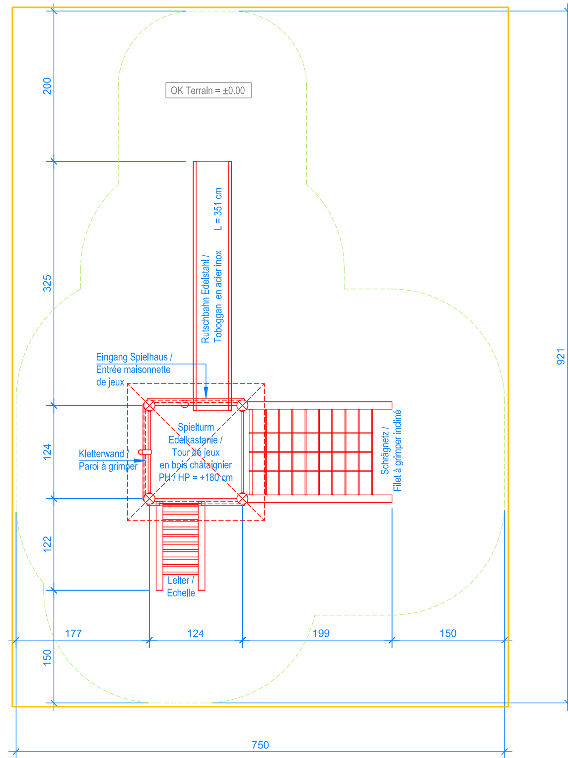
GRUNDRISS / PLAN 1:50
