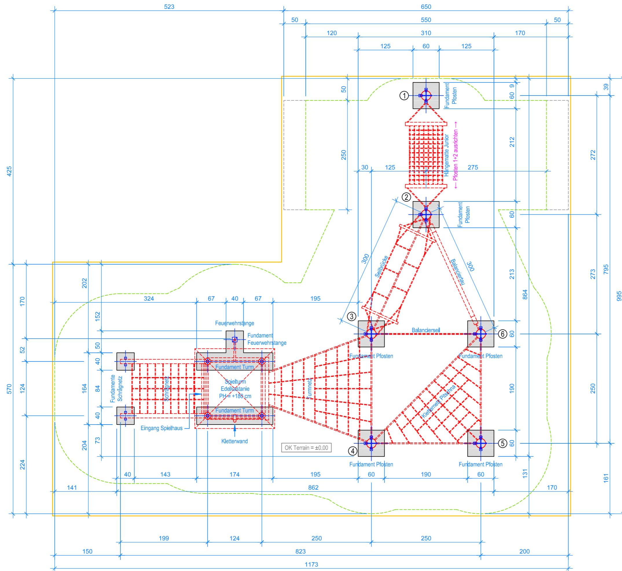
GRUNDRISS 1:50
