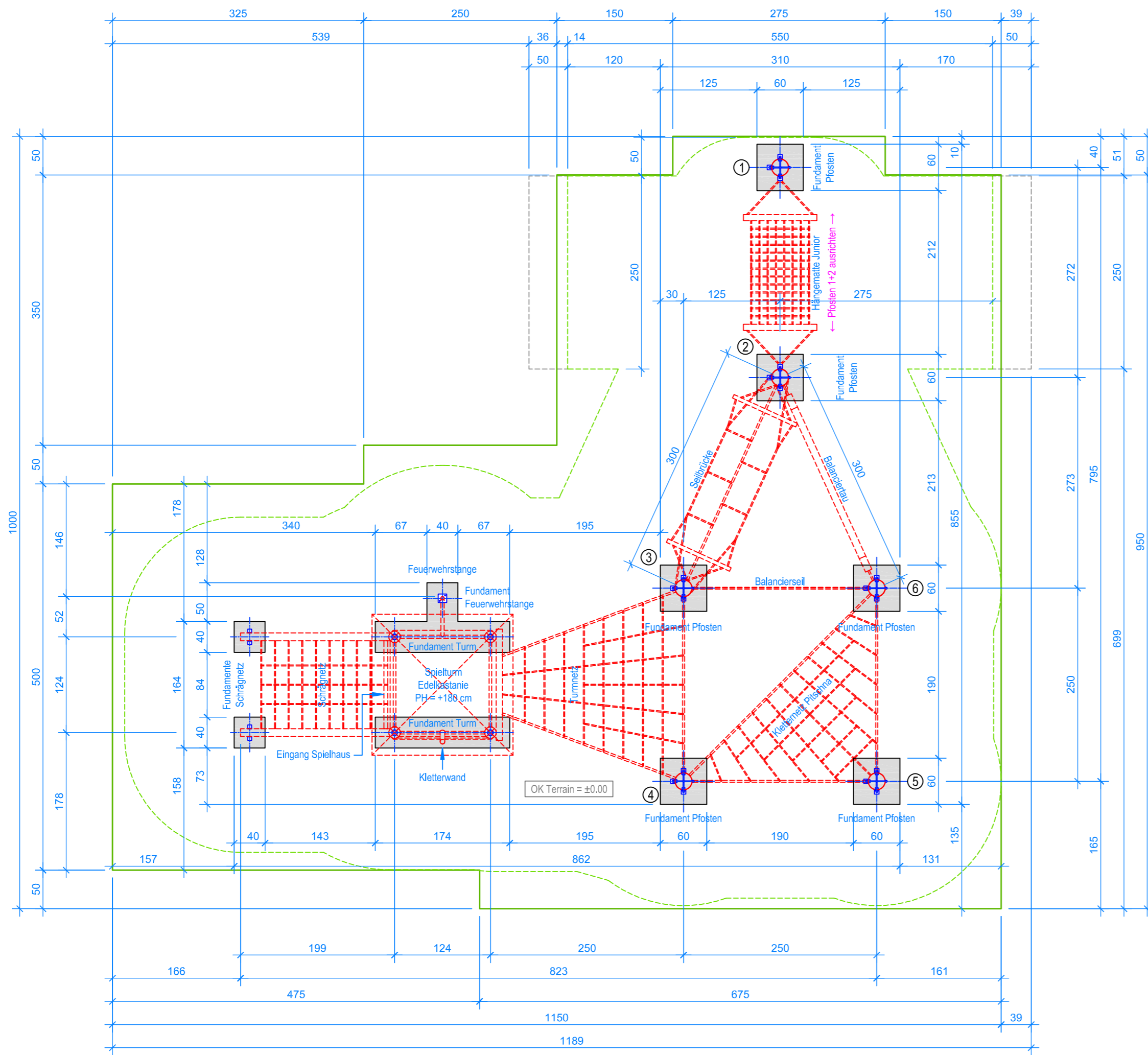
GRUNDRISS 1:50
