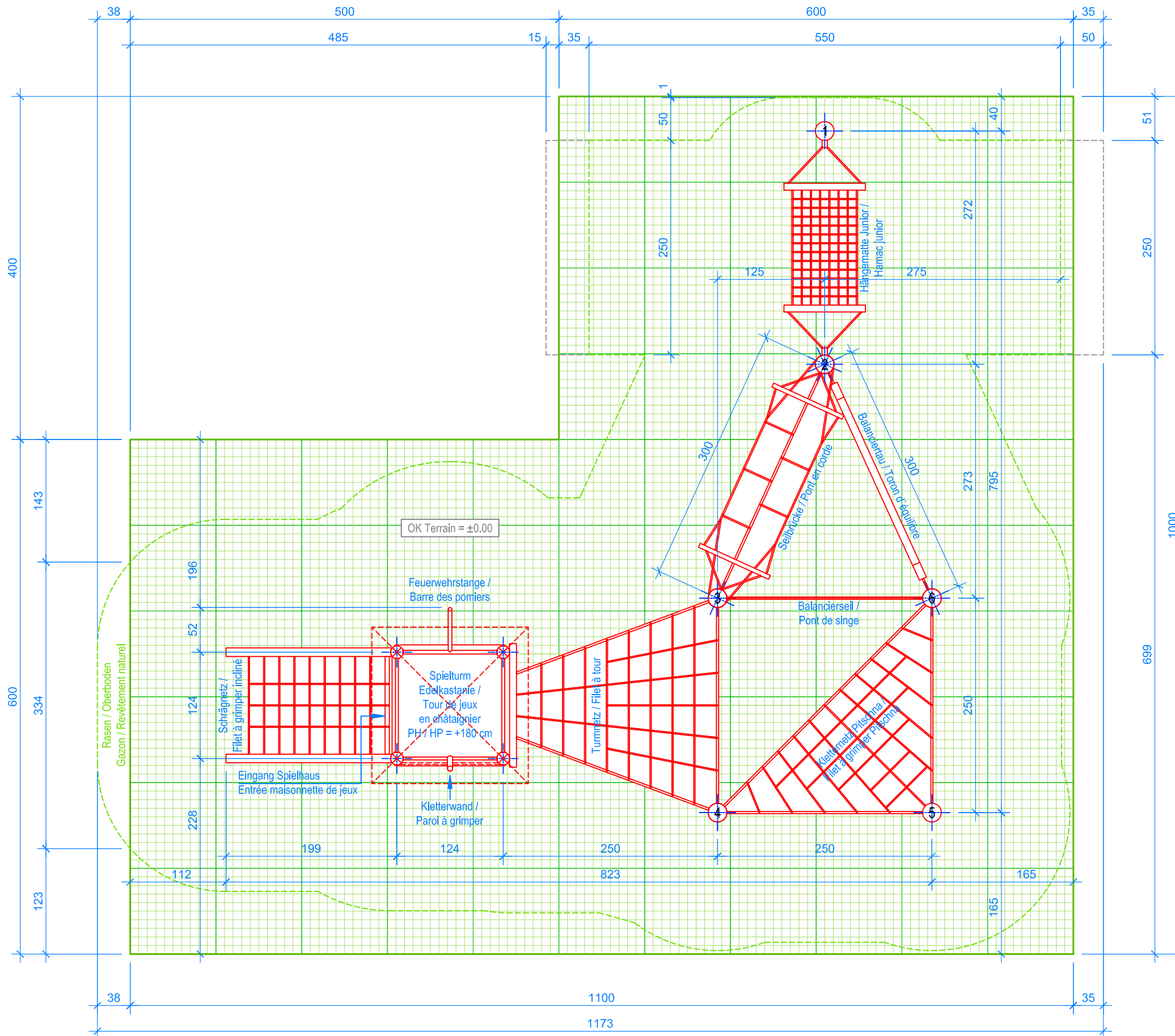
GRUNDRISS / PLAN 1:50
