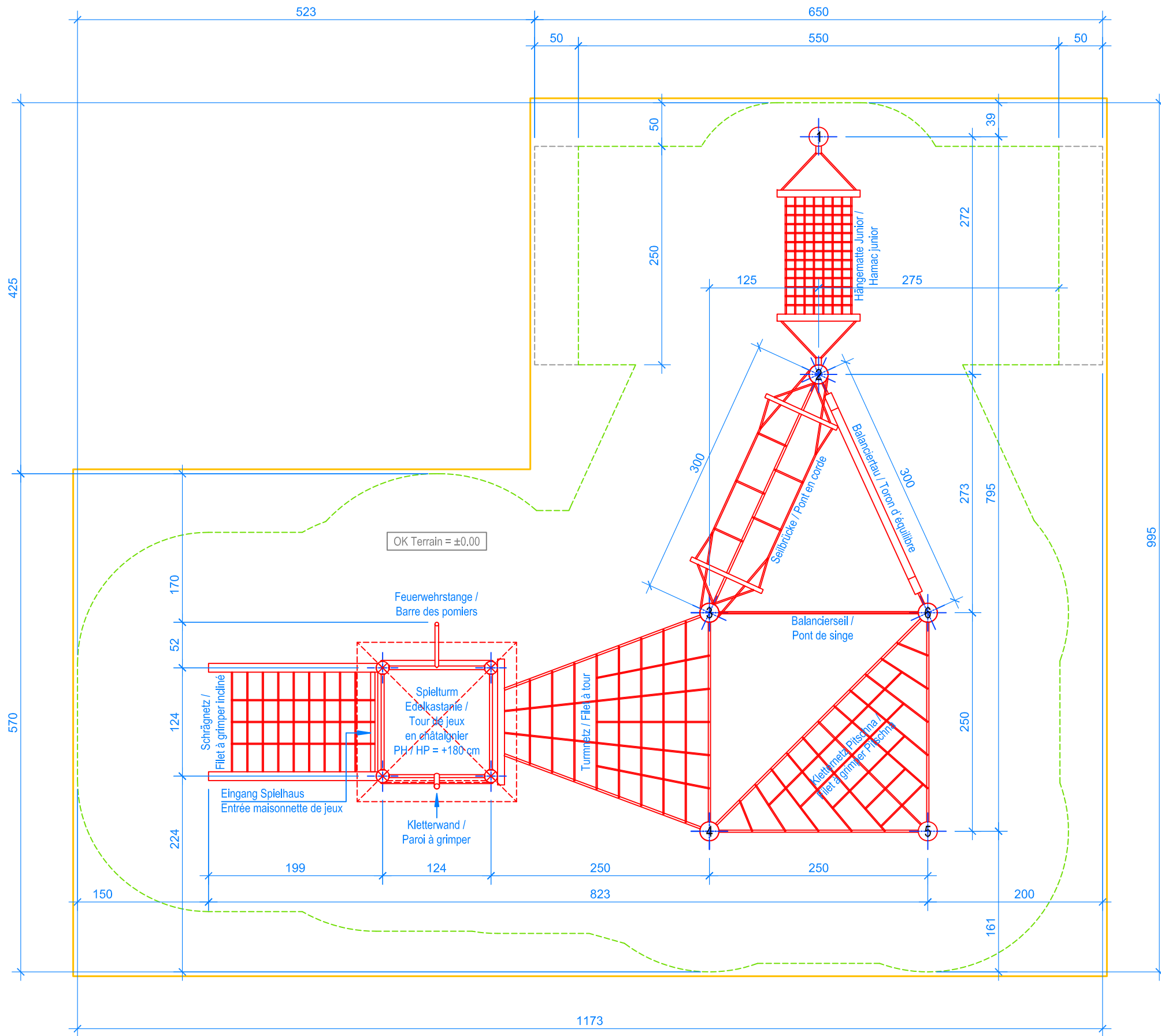
GRUNDRISS / PLAN 1:50
