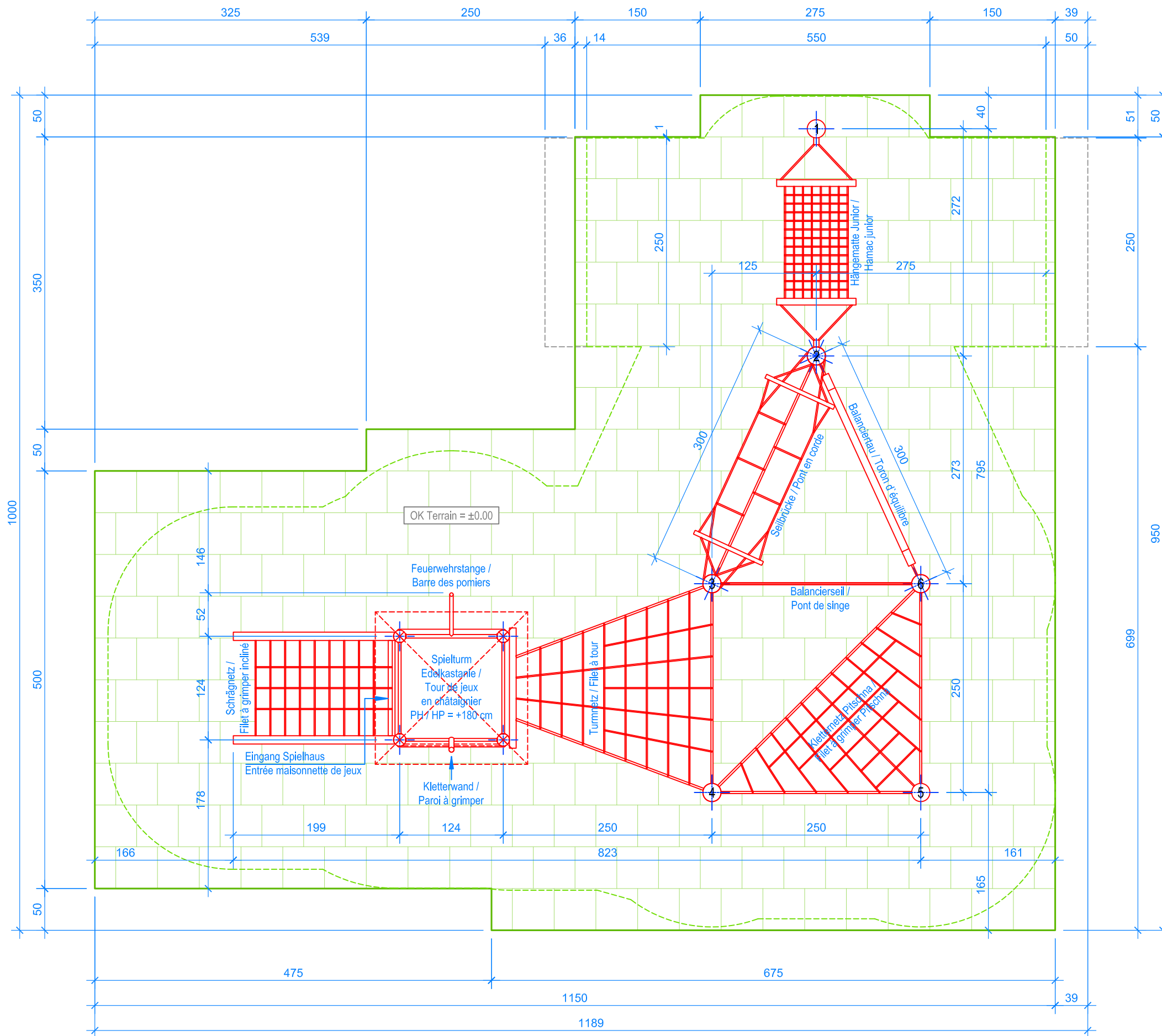
GRUNDRISS / PLAN 1:50
