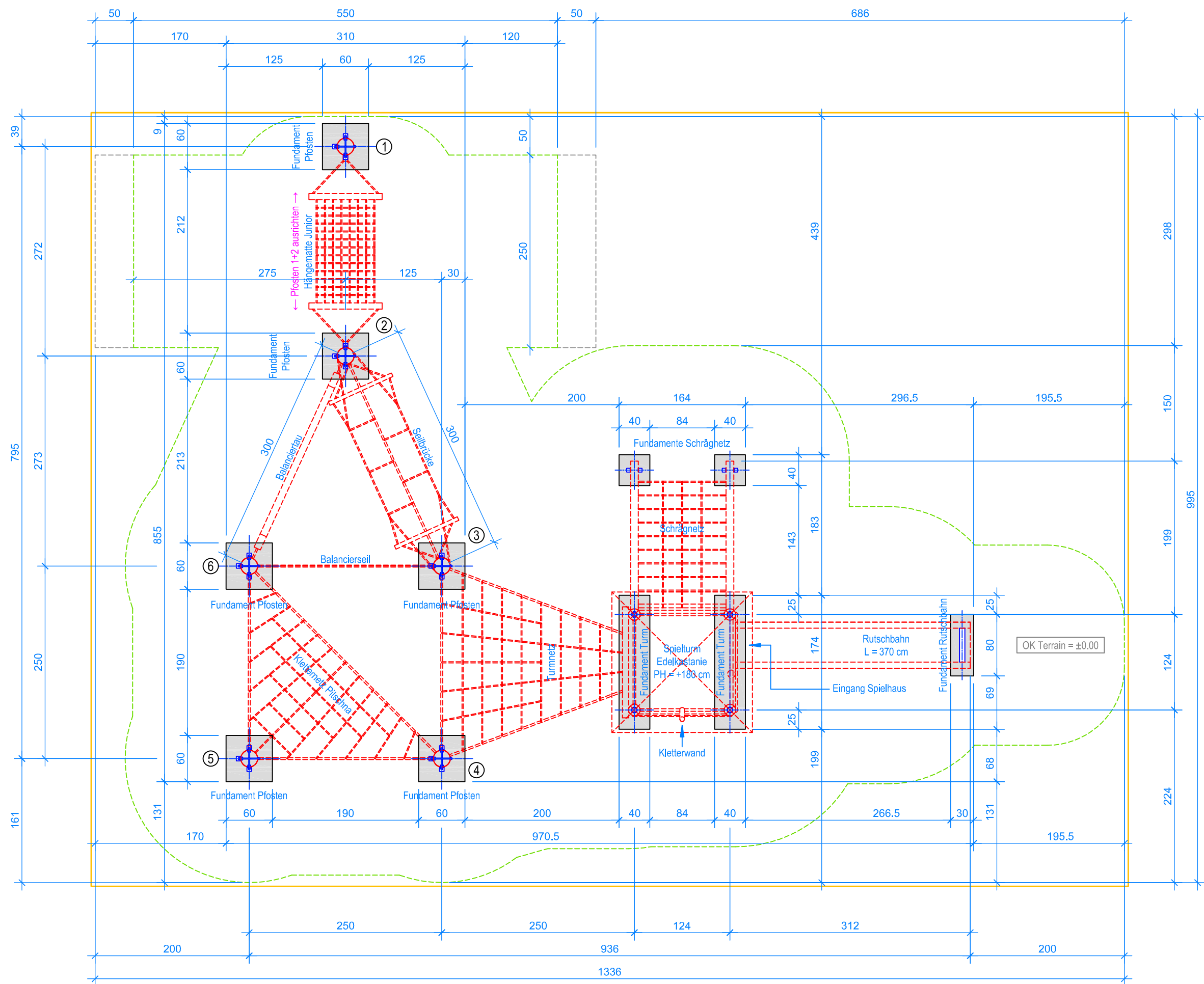
GRUNDRISS 1:50
