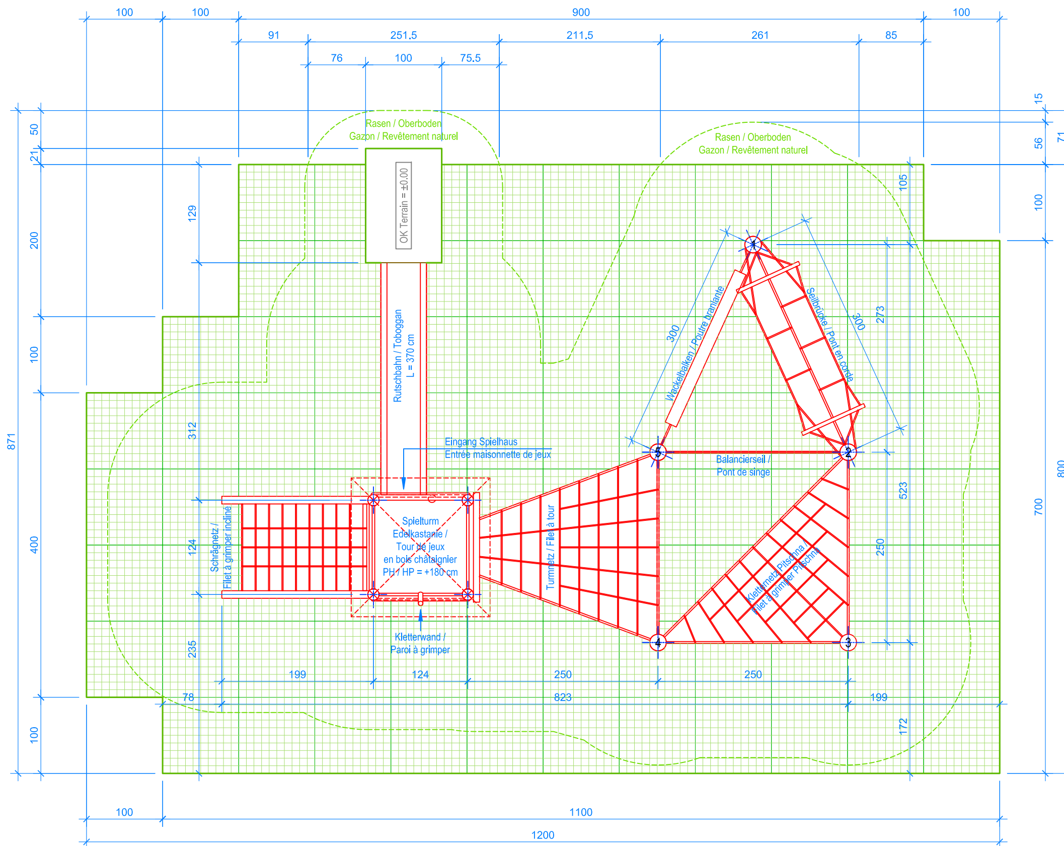
GRUNDRISS / PLAN 1:50
