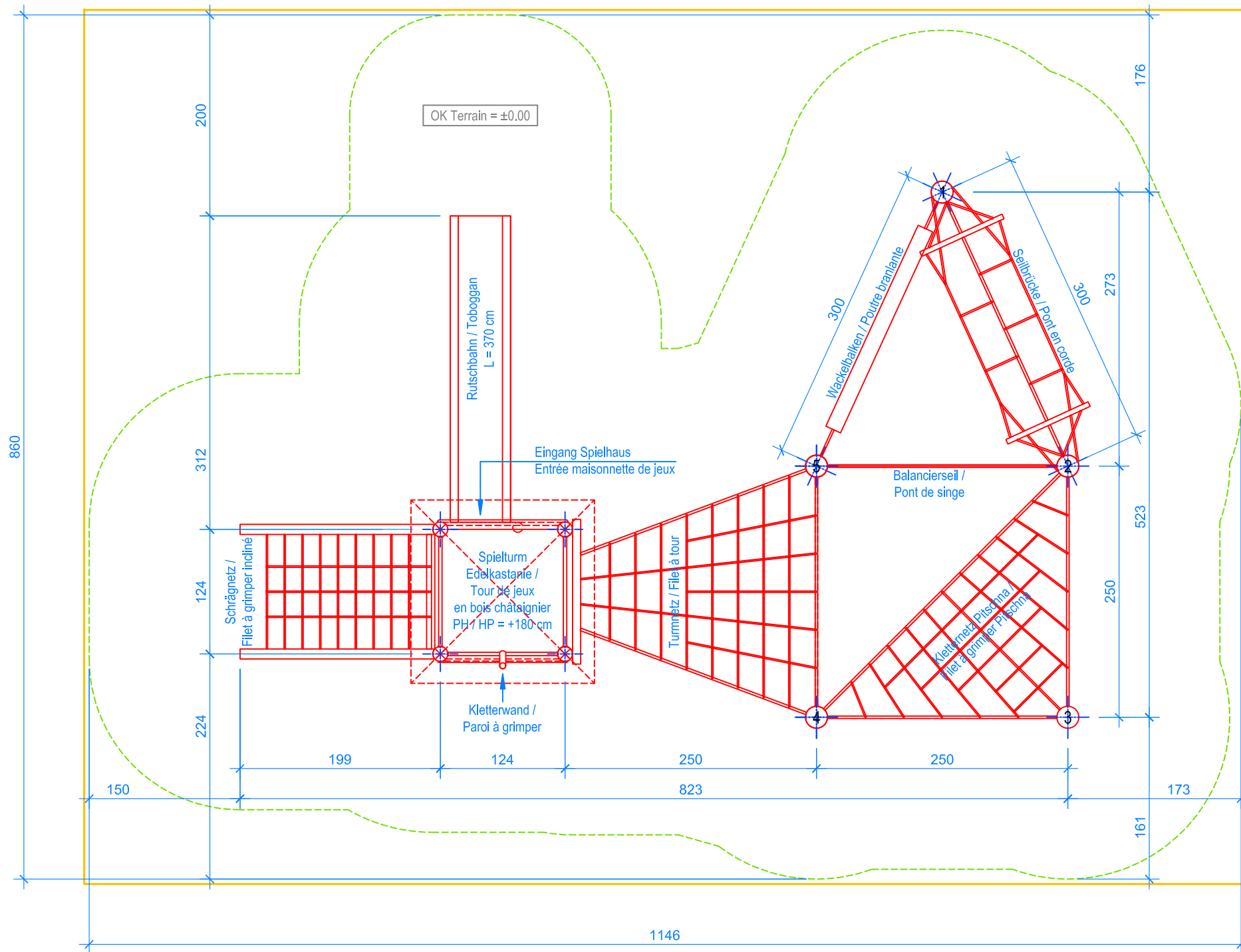
GRUNDRISS / PLAN 1:50
