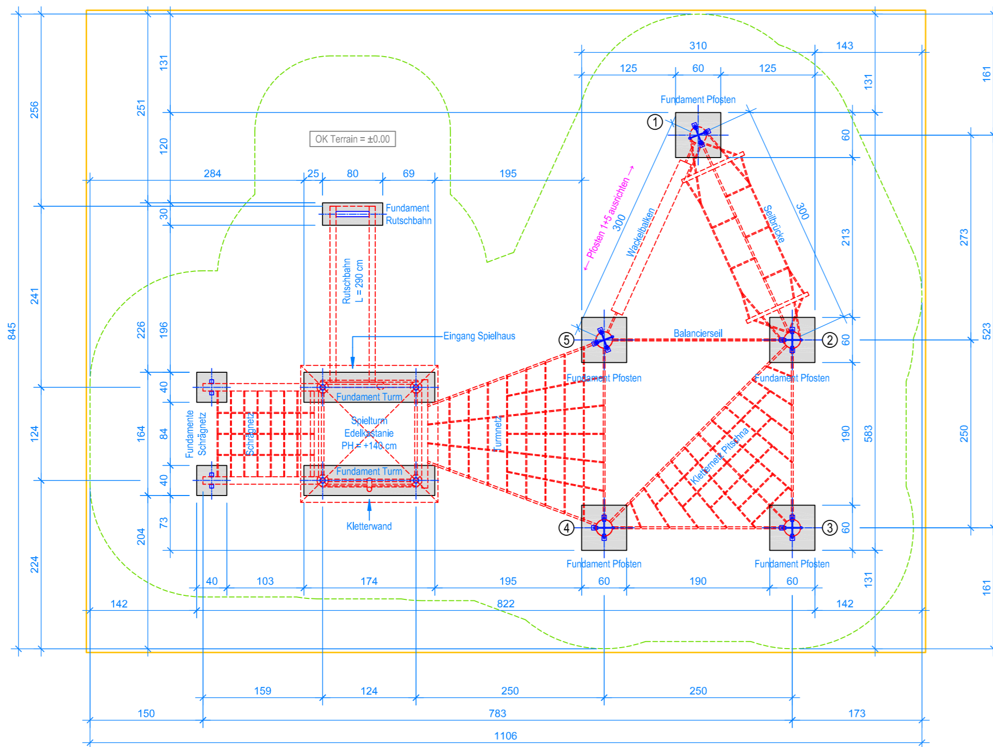
GRUNDRISS 1:50
