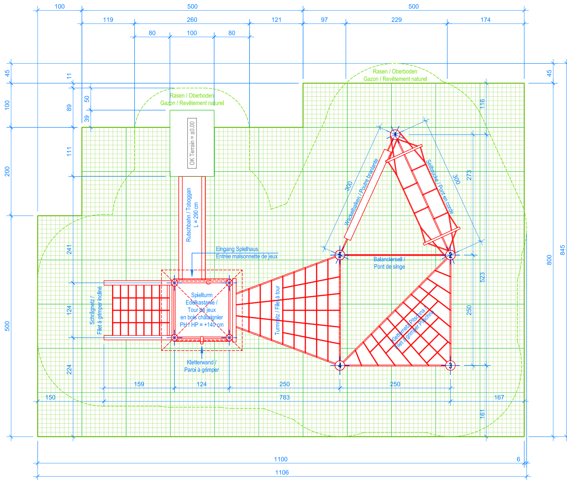
GRUNDRISS / PLAN 1:50
