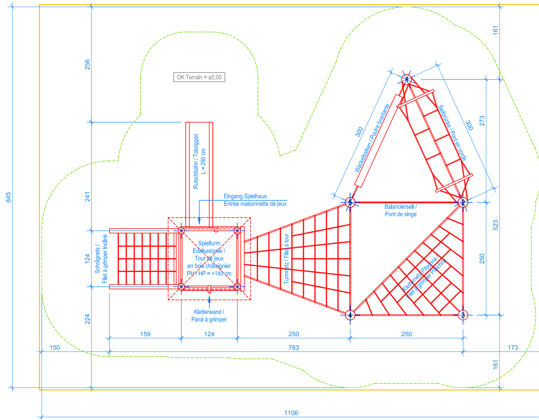
GRUNDRISS / PLAN 1:50
