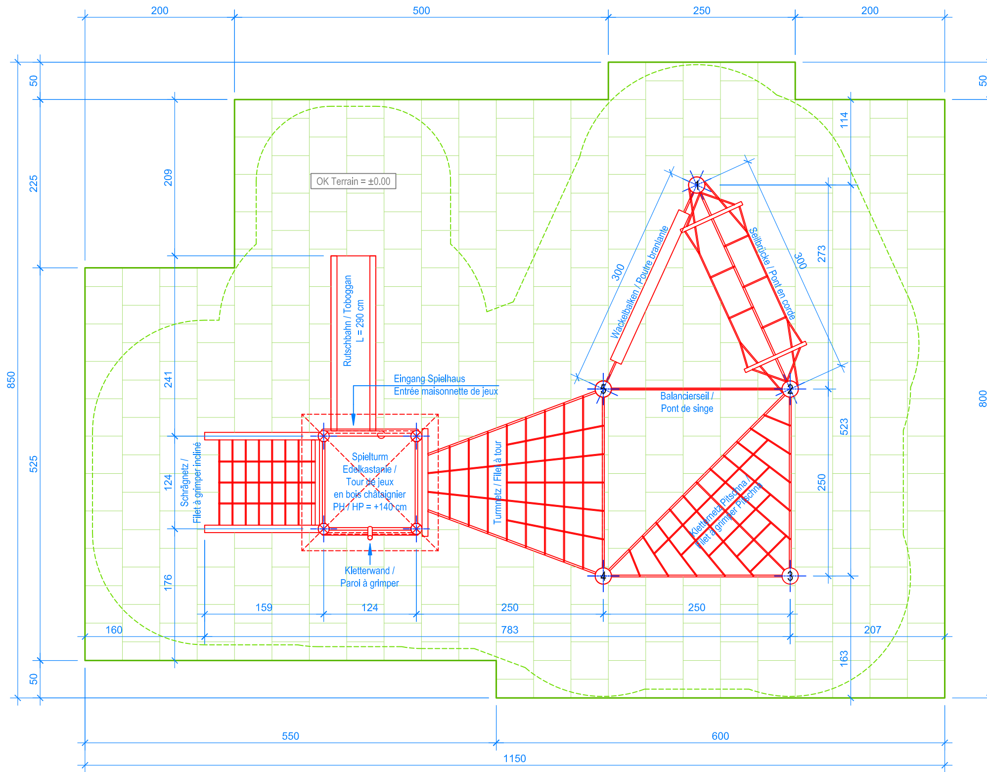
GRUNDRISS / PLAN 1:50
