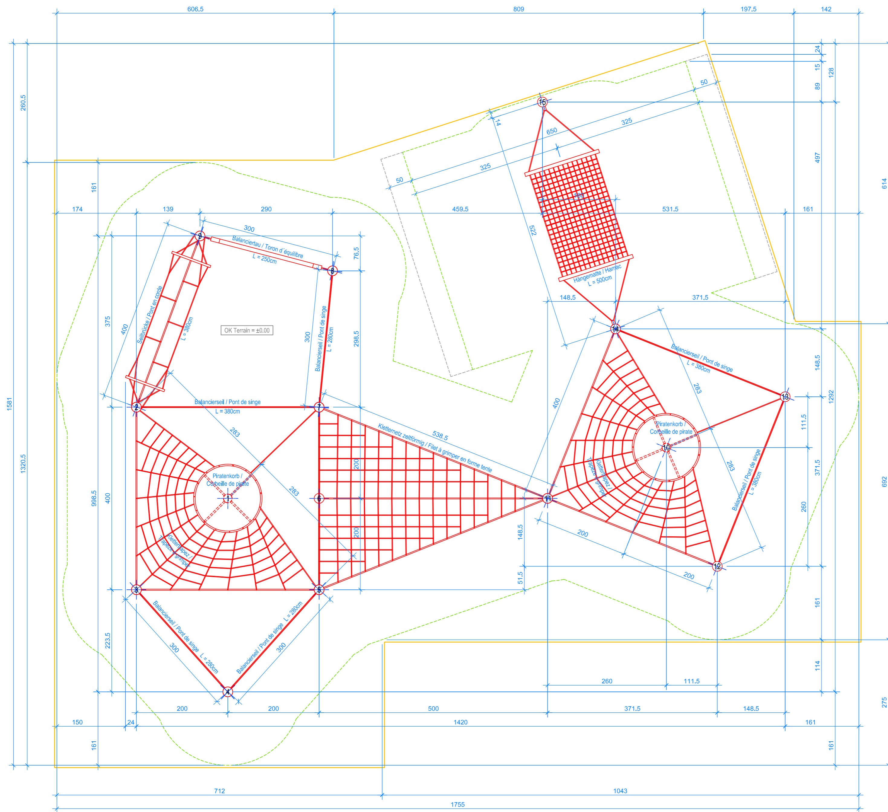
GRUNDRISS / PLAN 1:50
