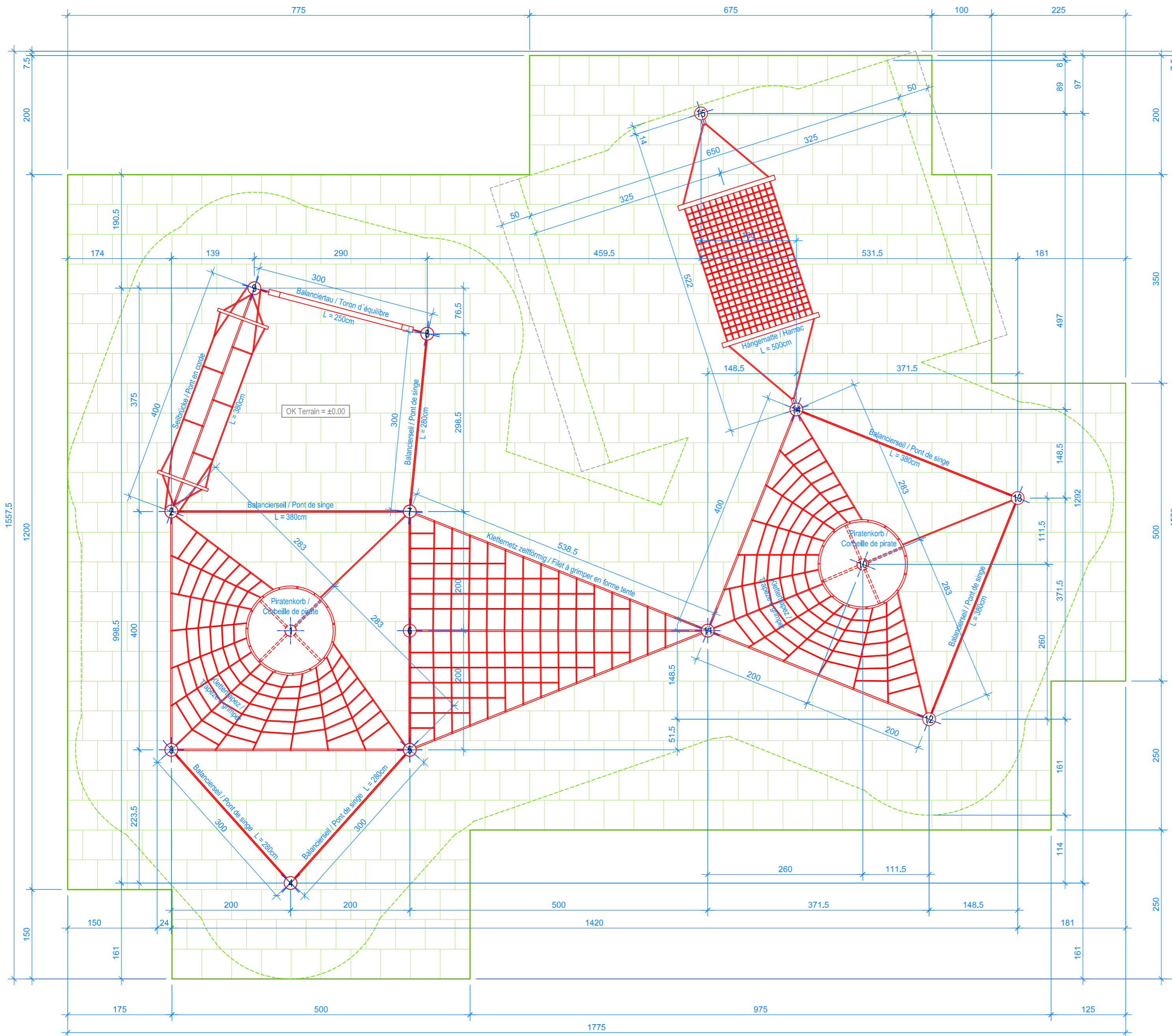
GRUNDRISS / PLAN 1:50
